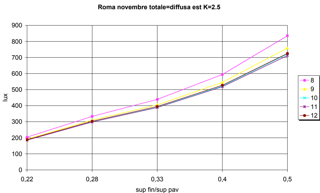
Figura 4.52. Roma, novembre, est, radiazione totale, K=2.5
