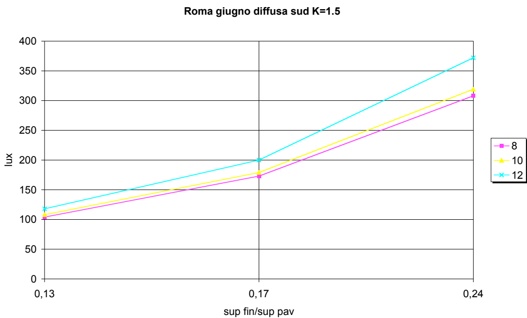
Figura 4.21. Roma, giugno, sud, radiazione diffusa, K=1.5
