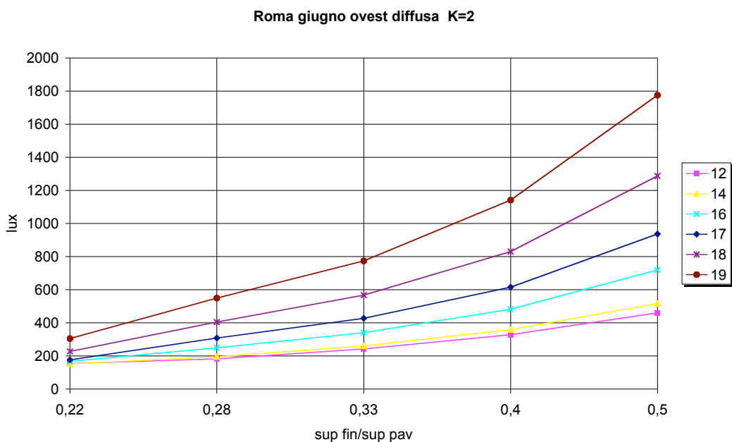
Figura 4.55. Roma, giugno, ovest, radiazione diffusa, K=2
