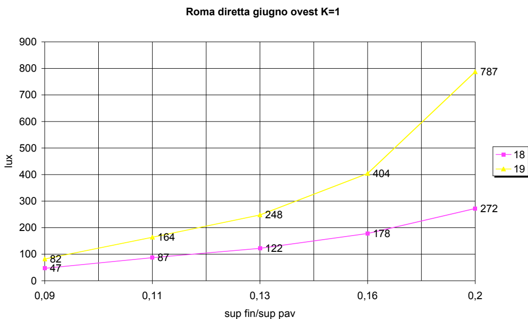
Figura 4.65. Roma, giugno, ovest, radiazione diretta, K=1
