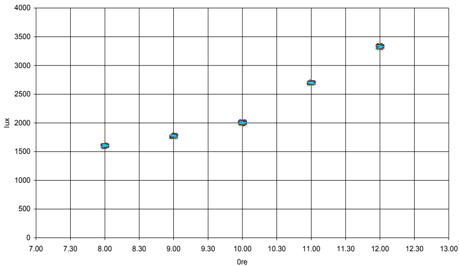
Figura 3.31. Roma, febbraio, radiazione totale, stanza 5x5, finestra 2x2
