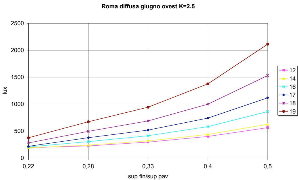
Figura 4.56. Roma, giugno, ovest, radiazione diffusa, K=2.5
