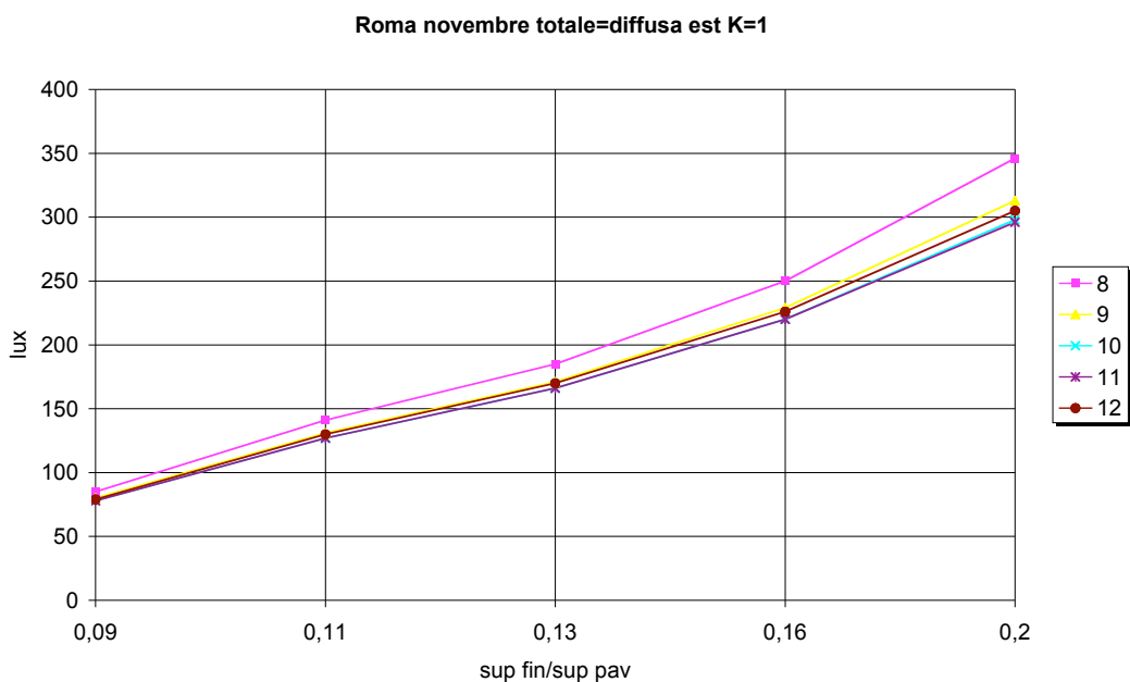
Figura 4.50. Roma, novembre, est, radiazione totale, K=1
