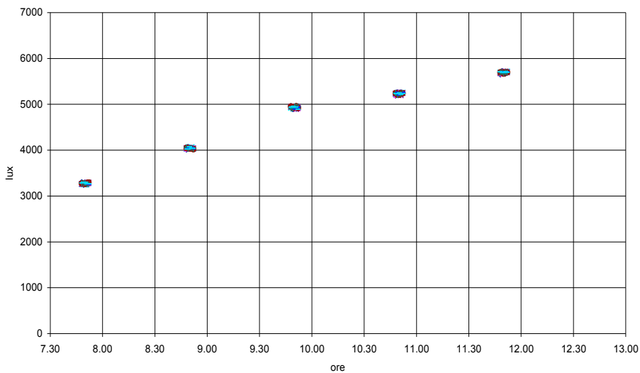
Figura 3.32. Roma, febbraio, radiazione totale, stanza 5x5, finestra 5x2
