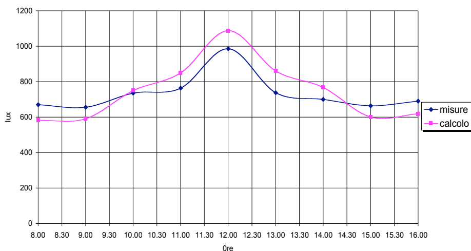
Figura 3.40. Roma, febbraio, est, radiazione totale, stanza 5x5, finestra 2x2
