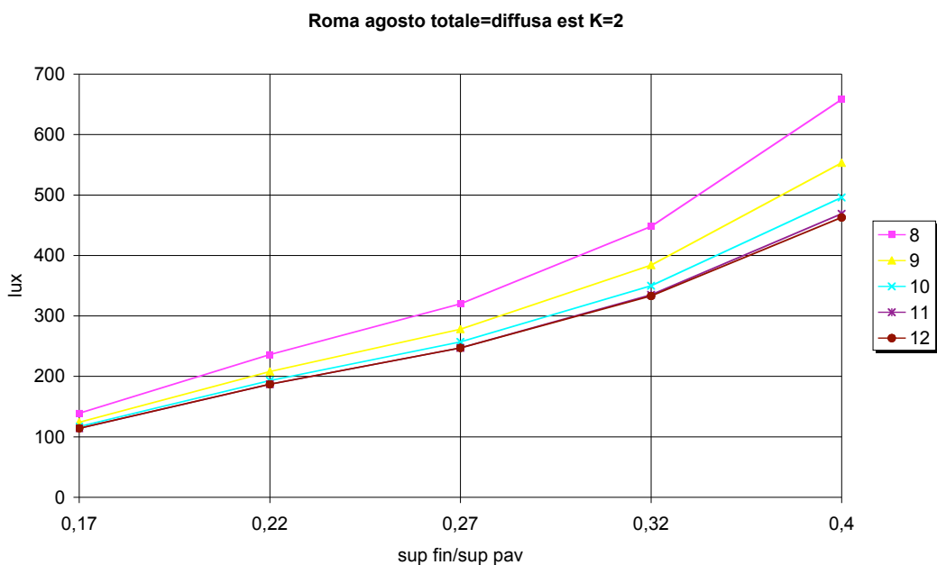
Figura 4.48. Roma, agosto, est, radiazione totale, K=2
