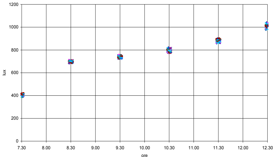
Figura 3.39. Roma, febbraio, radiazione totale, stanza 5x9, finestra 2x2
