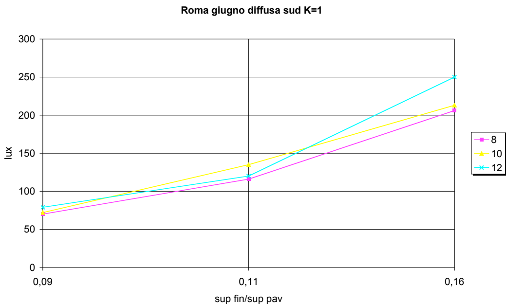
Figura 4.20. Roma, giugno, sud, radiazione diffusa, K=1
