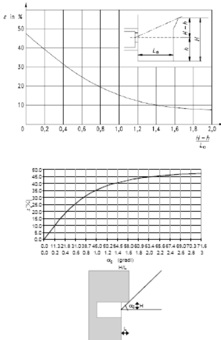
Figura 5.4. Calcolo del fattore finestra.
