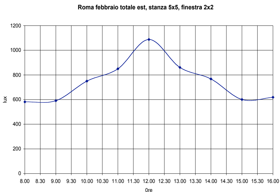
Figura 2.1. Esposizione Est, stanza 5x5, finestra 2x2
