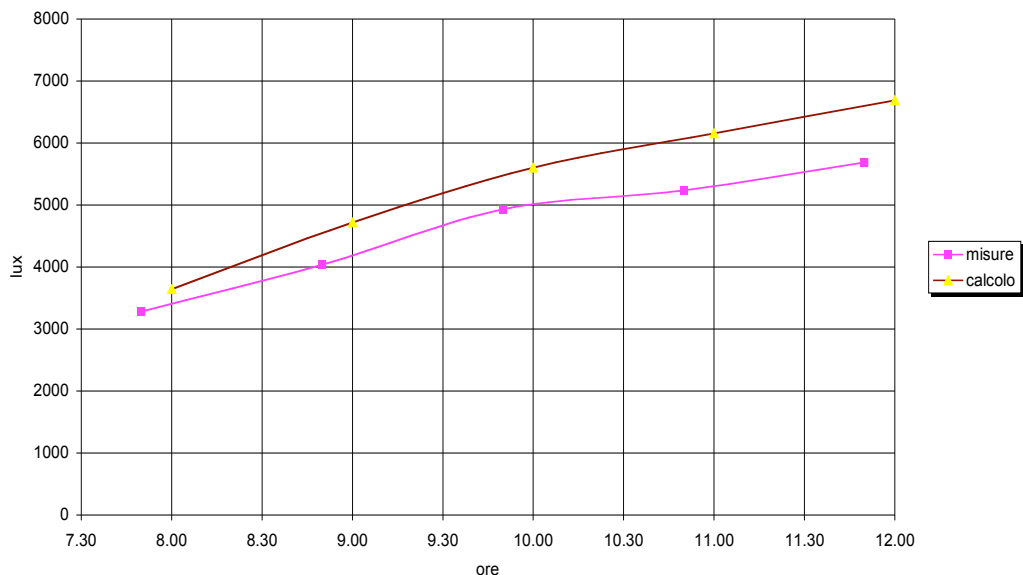
Figura 3.52. Roma, febbraio, sud, radiazione totale, stanza 5x5, finestra 5x2
