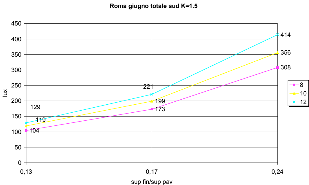
Figura 4.11. Roma, giugno, sud, radiazione totale, K=1.5
