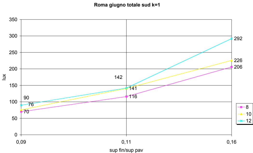
Figura 4.10. Roma, giugno, sud, radiazione totale, K=1
