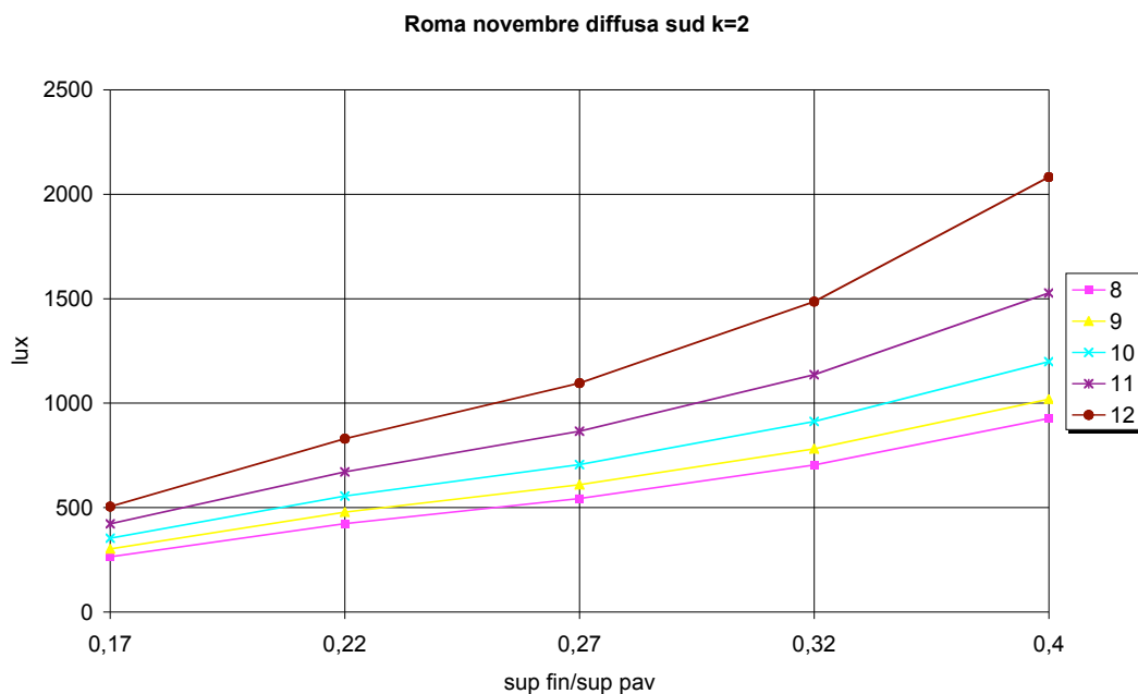
Figura 4.29. Roma, novembre, sud, radiazione diffusa, K=2
