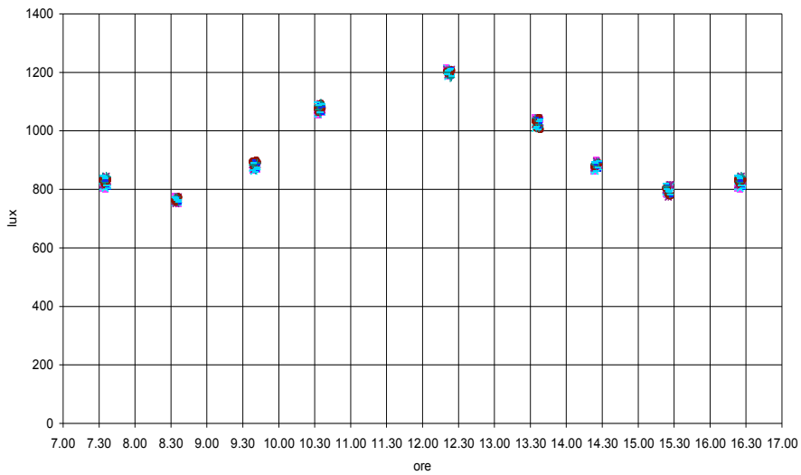
Figura 3.25. Roma, febbraio, radiazione totale, stanza 5x7, finestra 5x2
