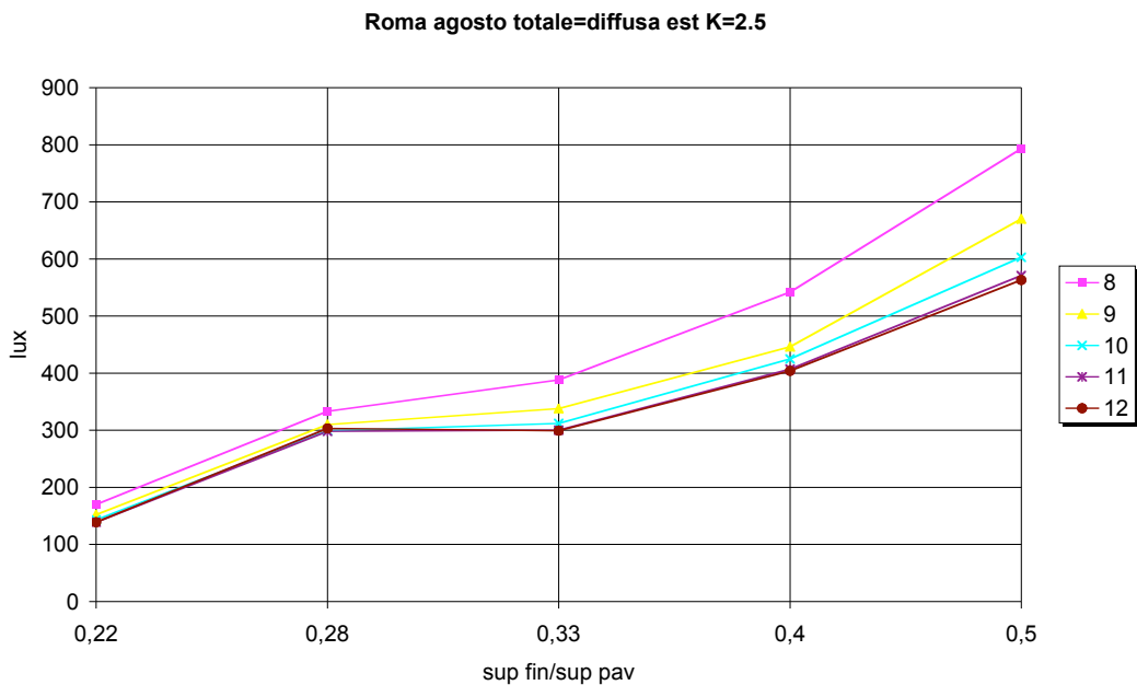
Figura 4.49. Roma, agosto, est, radiazione totale, K=2.5
