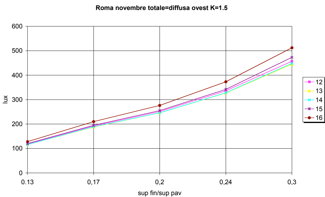
Figura 4.62. Roma, novembre, ovest, radiazione diffusa, K=1.5
