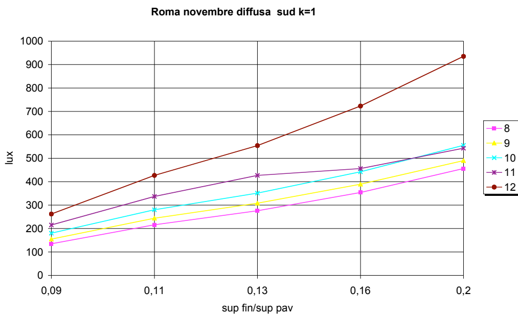
Figura 4.27. Roma, novembre, sud, radiazione diffusa, K=1
