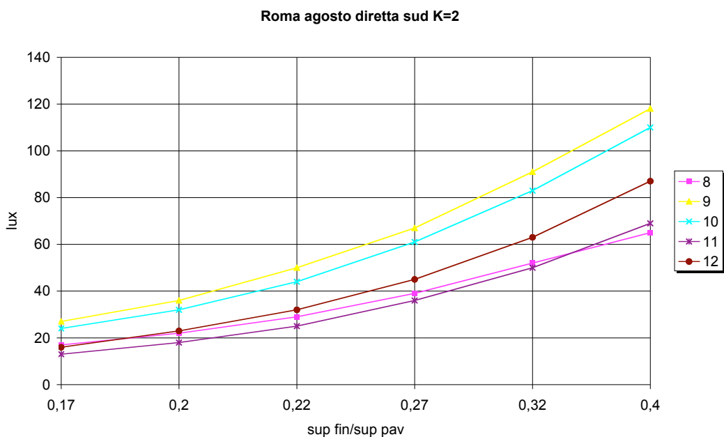
Figura 4.36. Roma, agosto, sud, radiazione diretta, K=2
