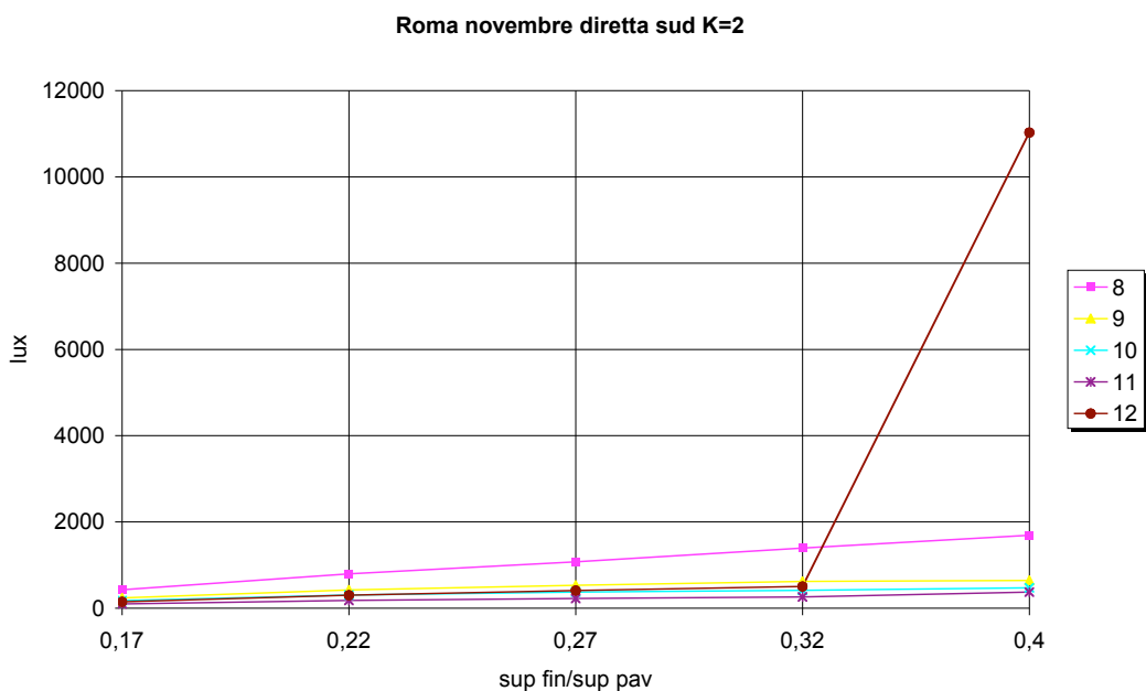
Figura 4.40. Roma, novembre, sud, radiazione diretta, K=2
