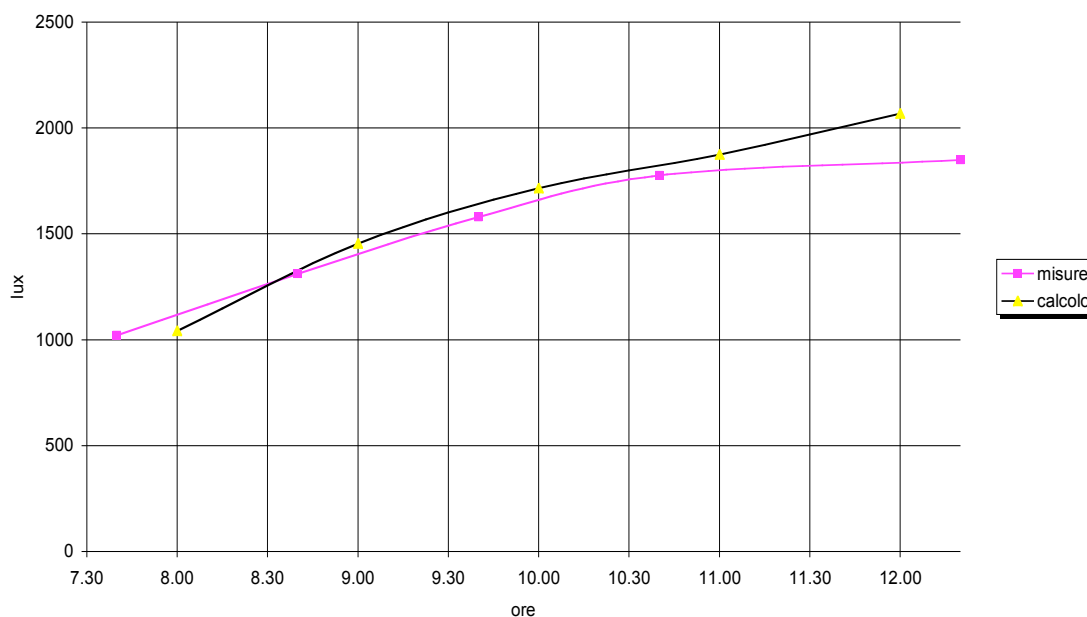
Figura 3.54. Roma, febbraio, sud, radiazione totale, stanza 5x7, finestra 3x2
