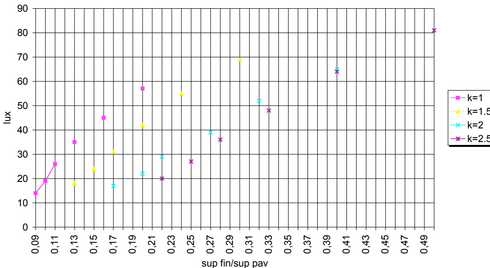
Figura 4.4. Roma, agosto, sud, radiazione diretta, ore 8
