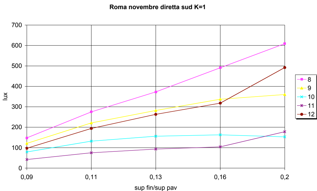
Figura 4.38. Roma, novembre, sud, radiazione diretta, K=1
