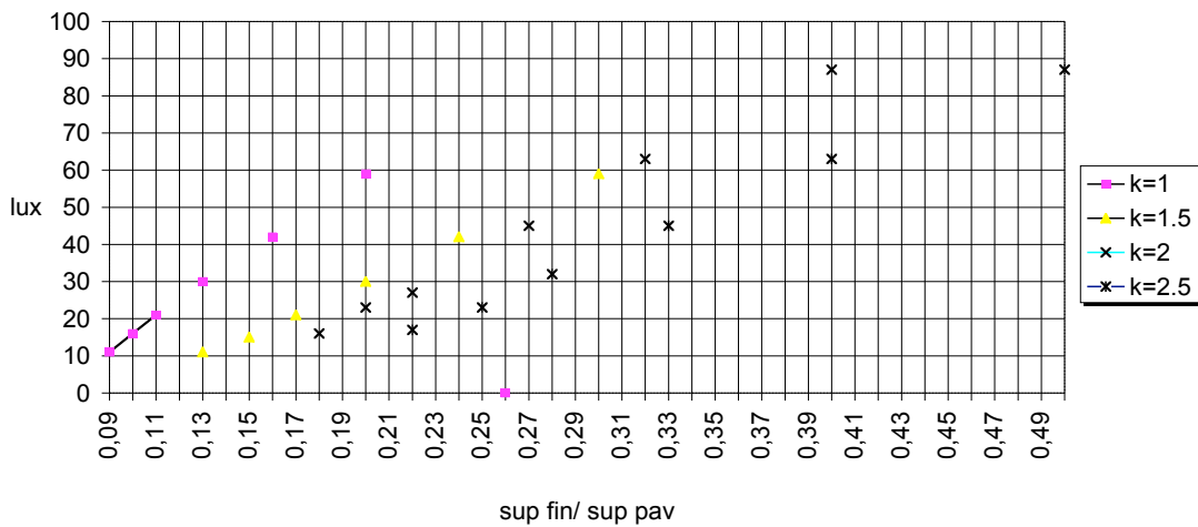
Figura 4.3. Roma, giugno, sud, radiazione diretta, ore 12
