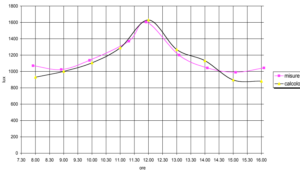
Figura 3.42. Roma, febbraio, est, radiazione totale, stanza 5x5, finestra 3x2
