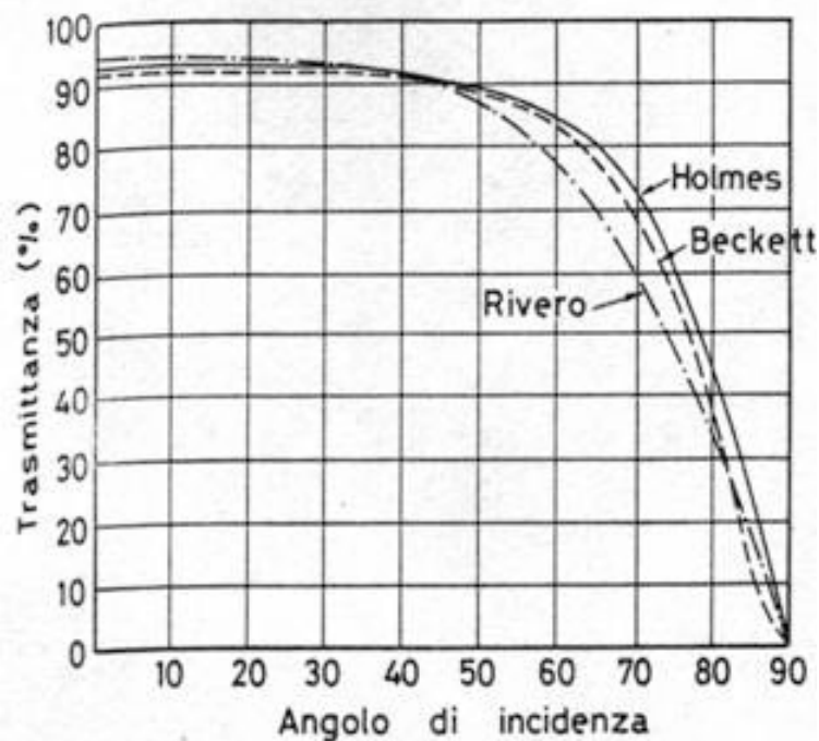
Figura 1.3. Curve relative alla trasmittanza di una lastra avente trasmittanza normale \tau_n=93\% in funzione degli angoli di incidenza della luce.
