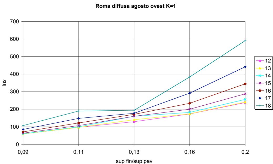
Figura 4.57. Roma, agosto, ovest, radiazione diffusa, K=1
