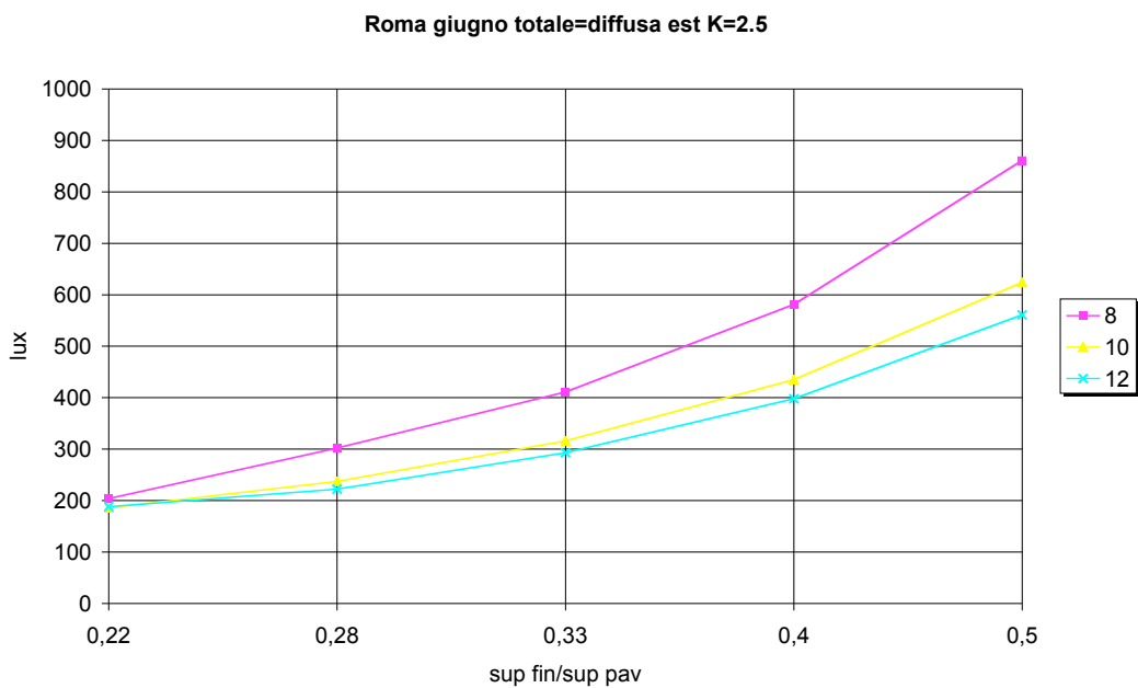
Figura 4.45. Roma, giugno, est, radiazione totale, K=2.5
