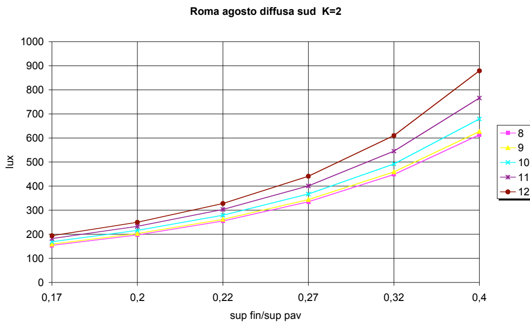
Figura 4.25. Roma, agosto, sud, radiazione diffusa, K=2
