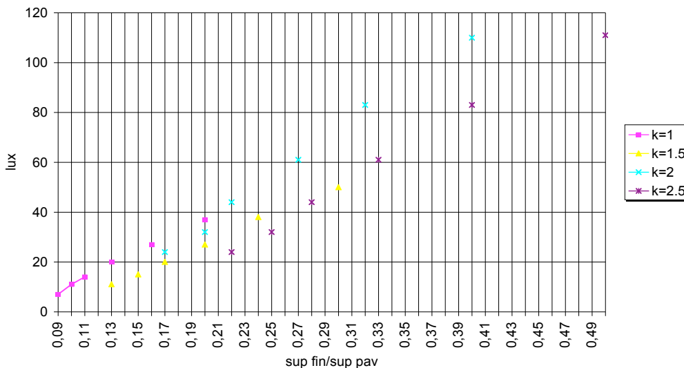
Figura 4.5. Roma, agosto, sud, radiazione diretta, ore 10
