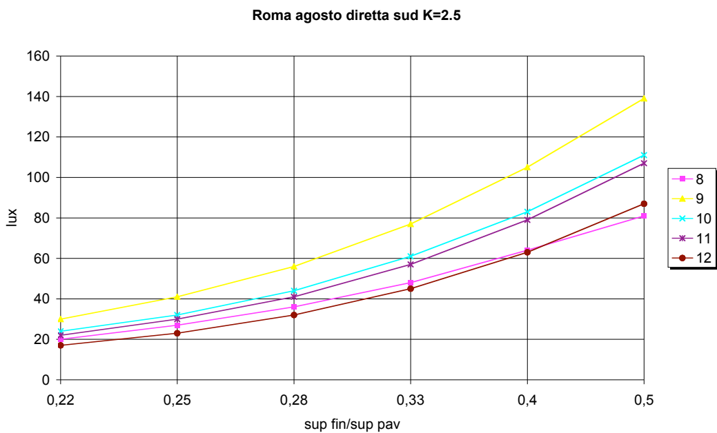
Figura 4.37. Roma, agosto, sud, radiazione diretta, K=2.5
