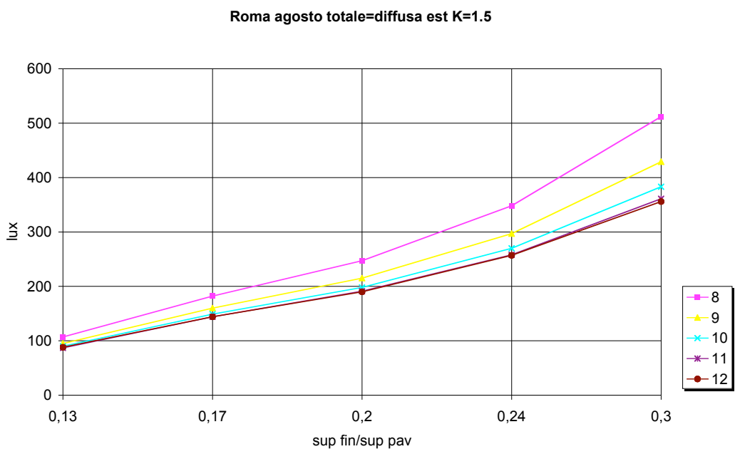
Figura 4.47. Roma, agosto, est, radiazione totale, K=1.5
