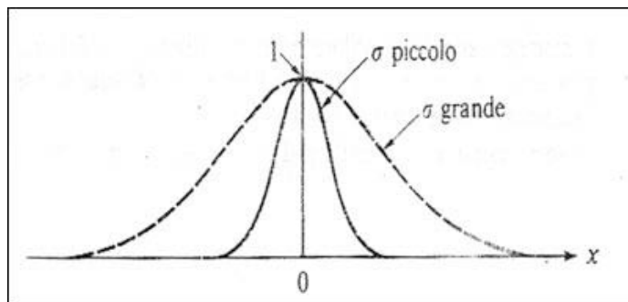
Figura 3.21. Funzione di Gauss a campana centrata su x=0
