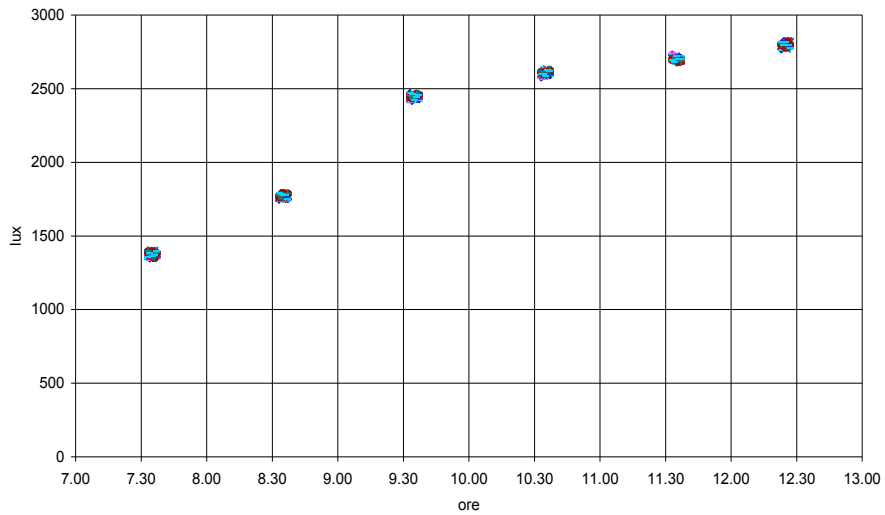
Figura 3.37. Roma, febbraio, radiazione totale, stanza 5x7, finestra 5x2
