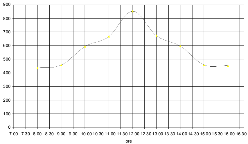
Figura 2.9. Esposizione Est, stanza 5x9, finestra 5x2
