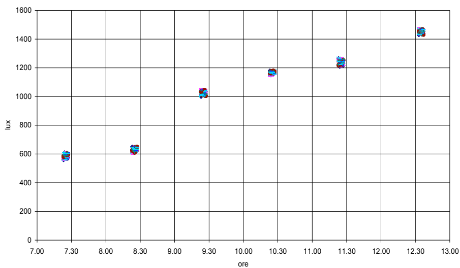
Figura 3.38. Roma, febbraio, radiazione totale, stanza 5x9, finestra 3x2
