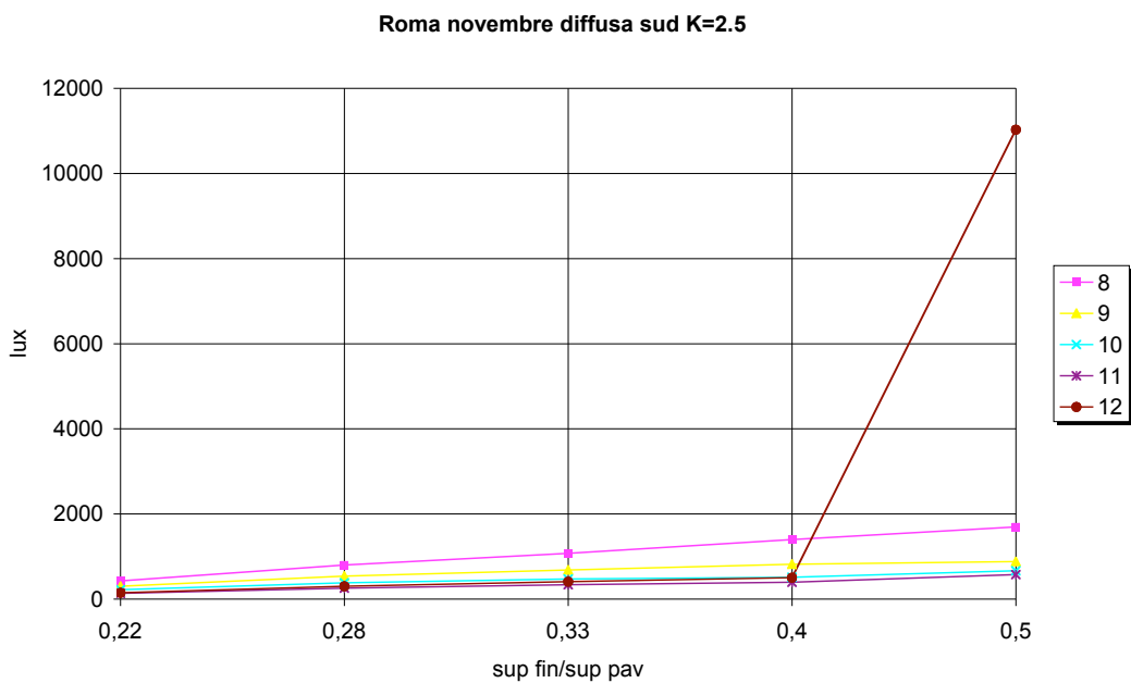
Figura 4.41. Roma, novembre, sud, radiazione diretta, K=2.5
