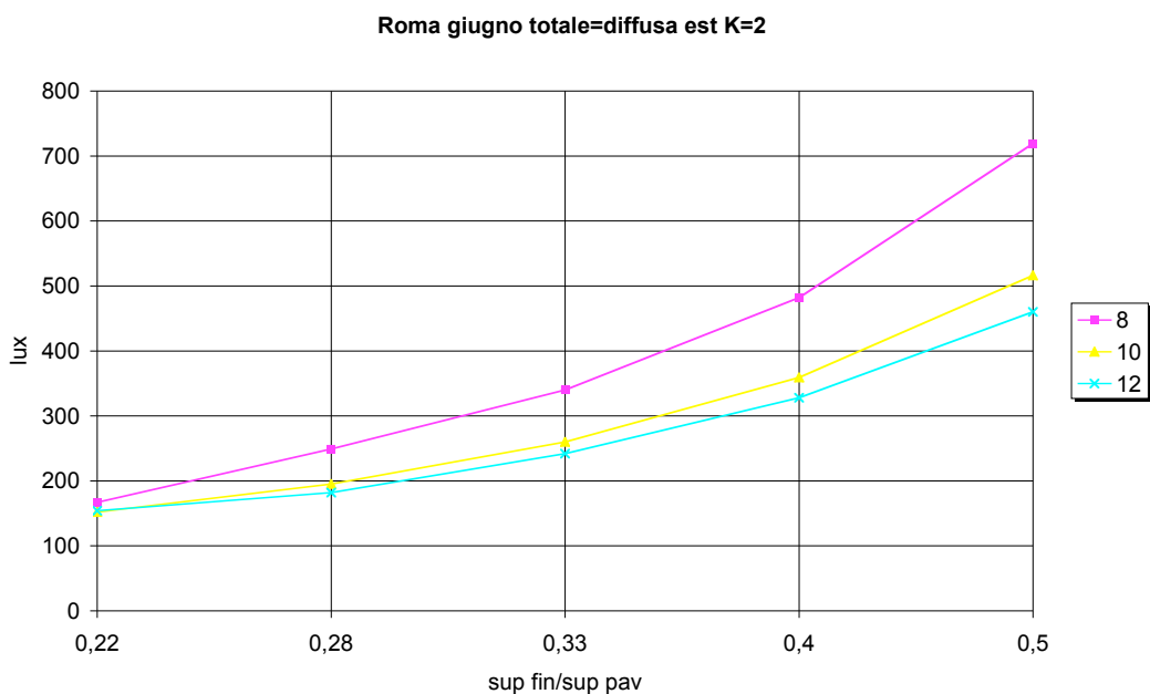
Figura 4.44. Roma, giugno, est, radiazione totale, K=2
