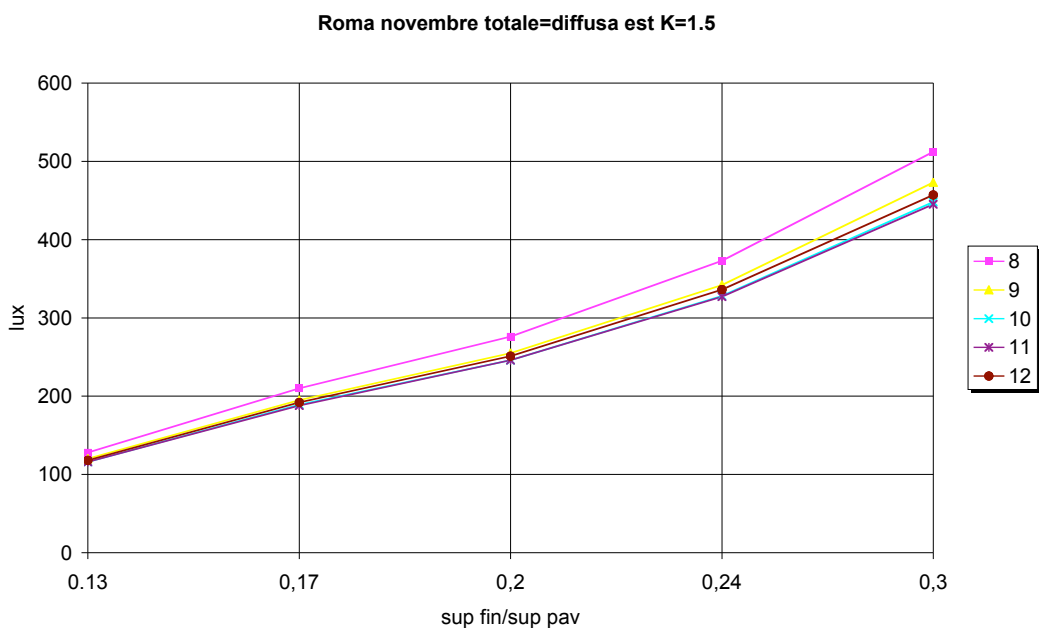
Figura 4.51. Roma, novembre, est, radiazione totale, K=1.5
