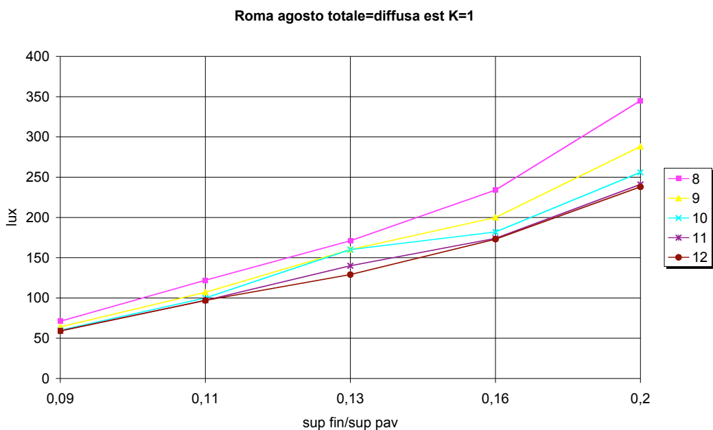
Figura 4.46. Roma, agosto, est, radiazione totale, K=1
