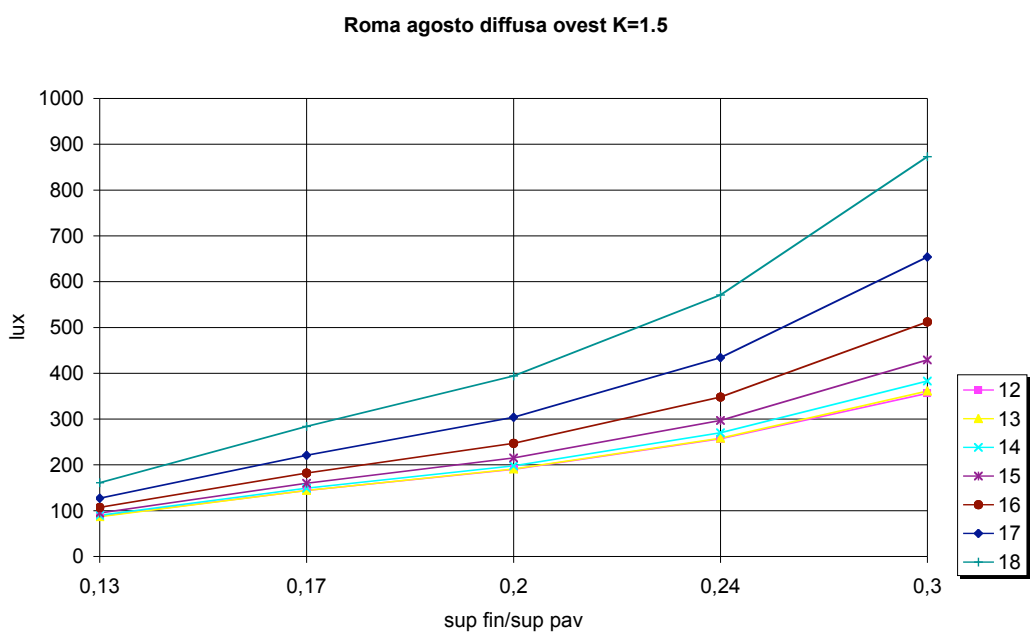
Figura 4.58. Roma, agosto, ovest, radiazione diffusa, K=1.5
