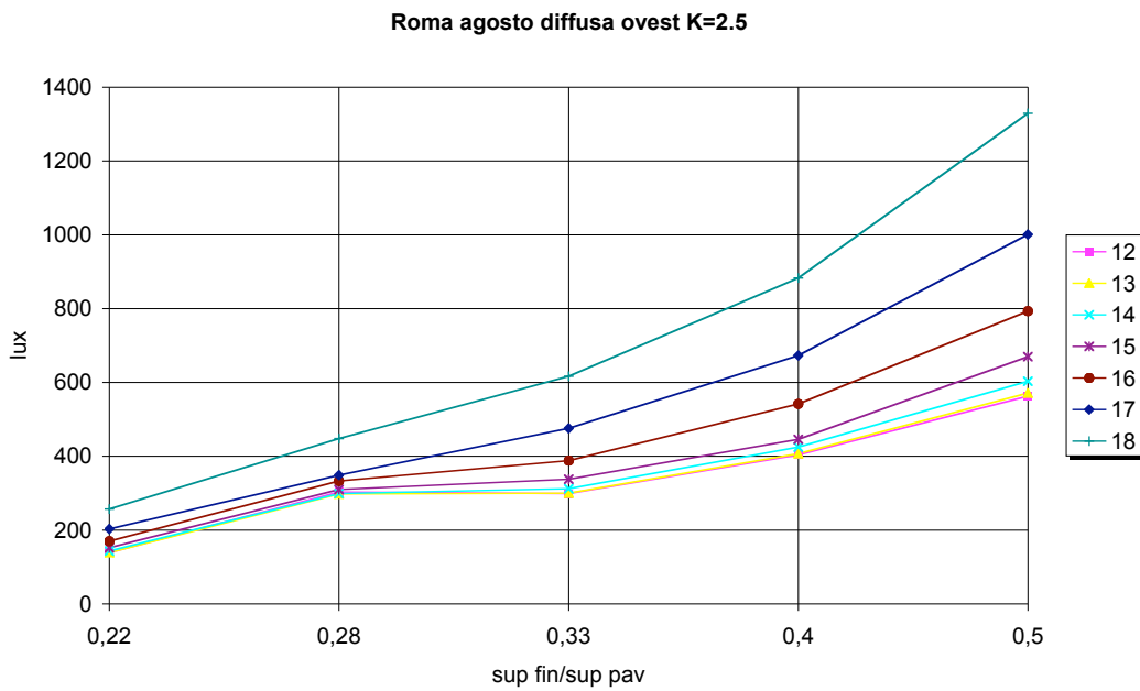
Figura 4.60. Roma, agosto, ovest, radiazione diffusa, K=2.5
