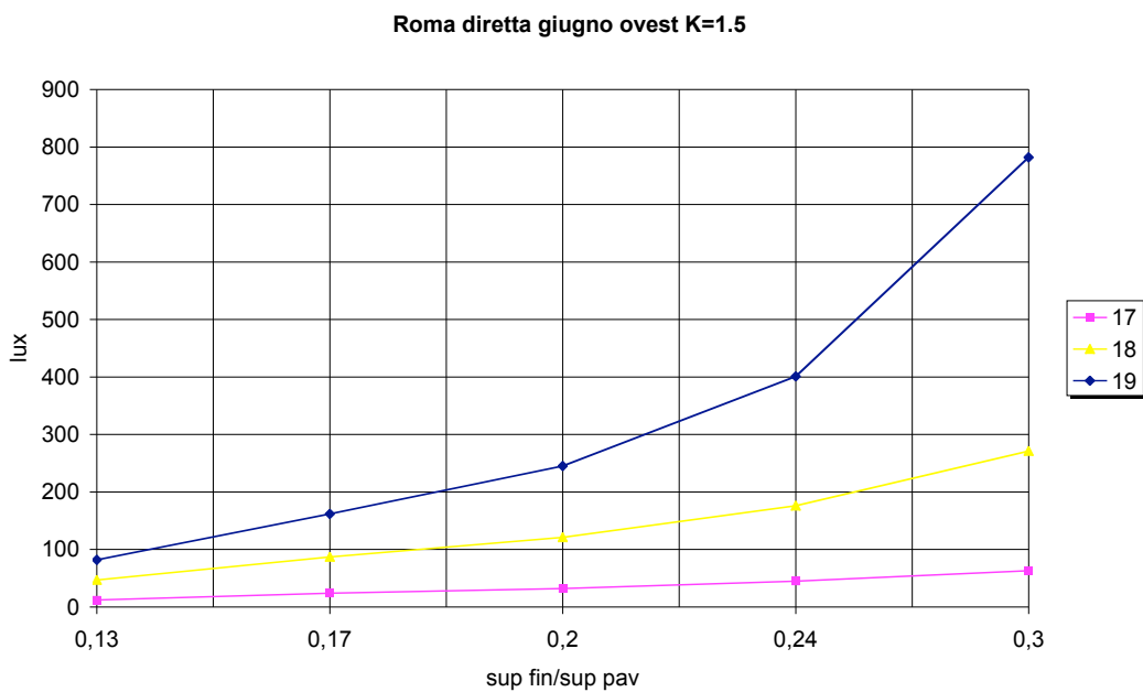
Figura 4.66. Roma, giugno, ovest, radiazione diretta, K=1.5
