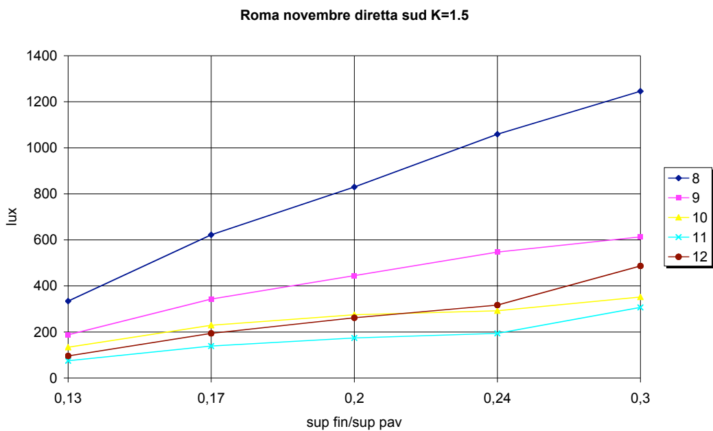
Figura 4.39. Roma, novembre, sud, radiazione diretta, K=1.5
