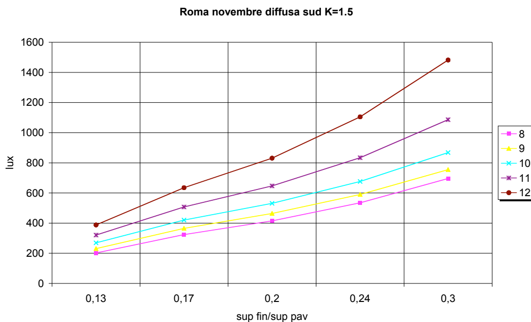
Figura 4.28. Roma, novembre, sud, radiazione diffusa, K=1.5
