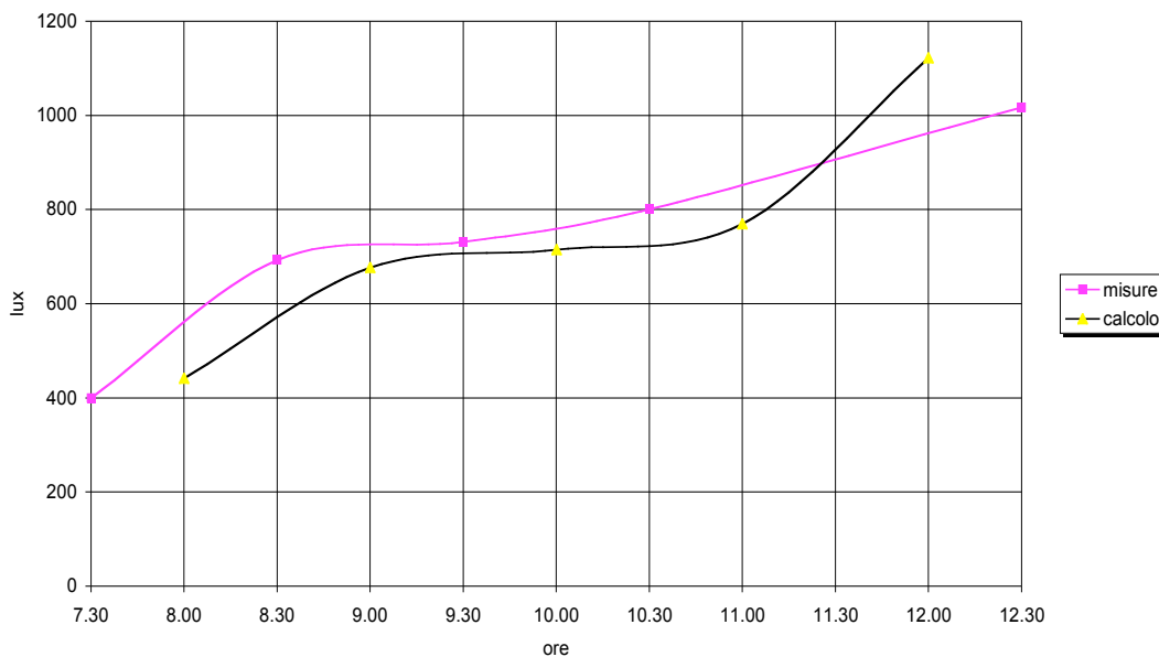
Figura 3.55. Roma, febbraio, sud, radiazione totale, stanza 5x9, finestra 2x2
