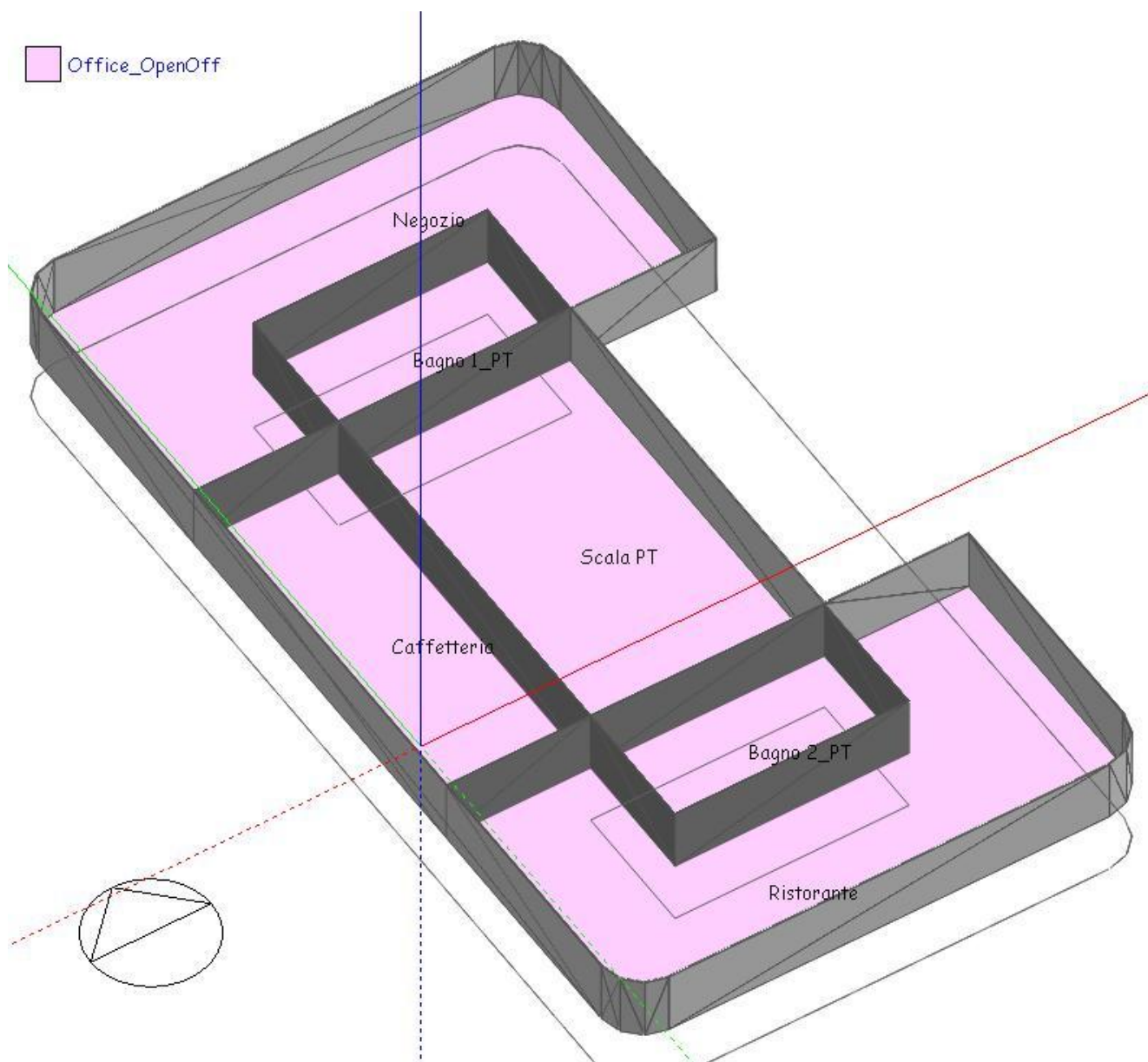
Figura 3.2.6– Vista assometrica del piano terreno.
