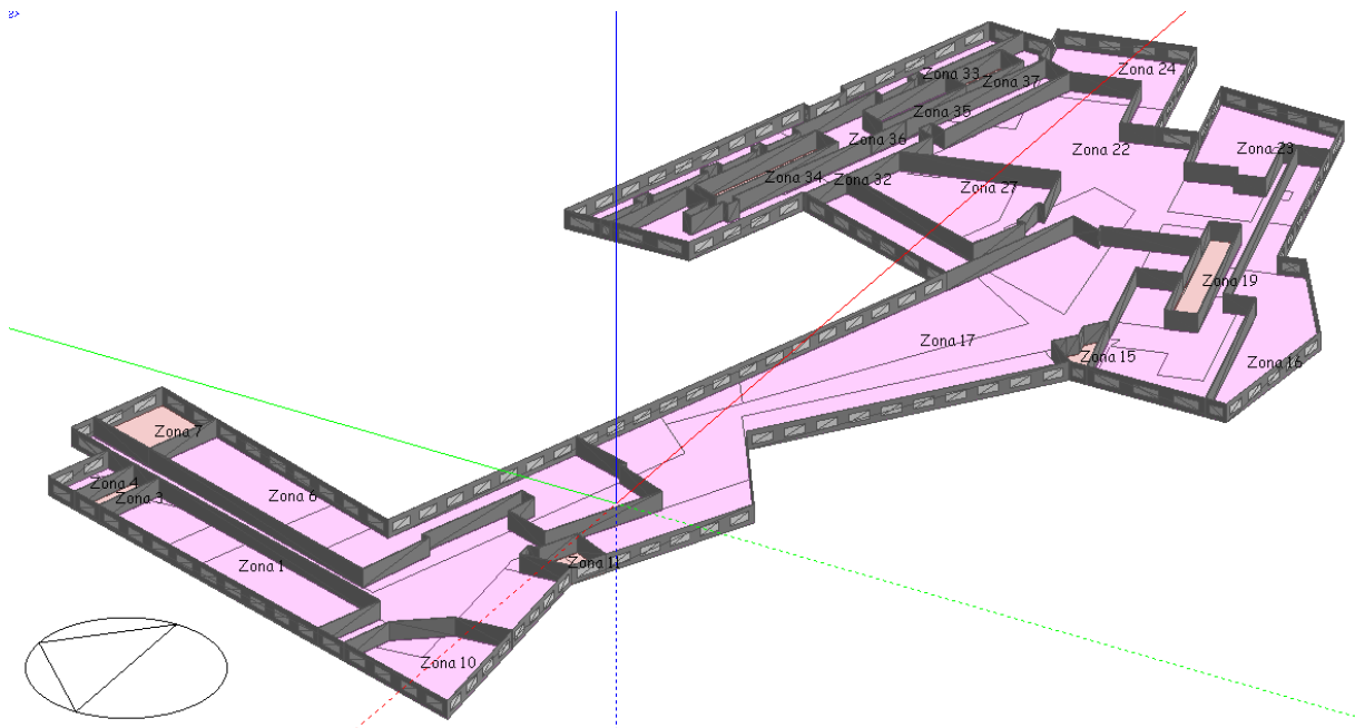
Figura 3.3.5 – Assonometria del secondo piano.
