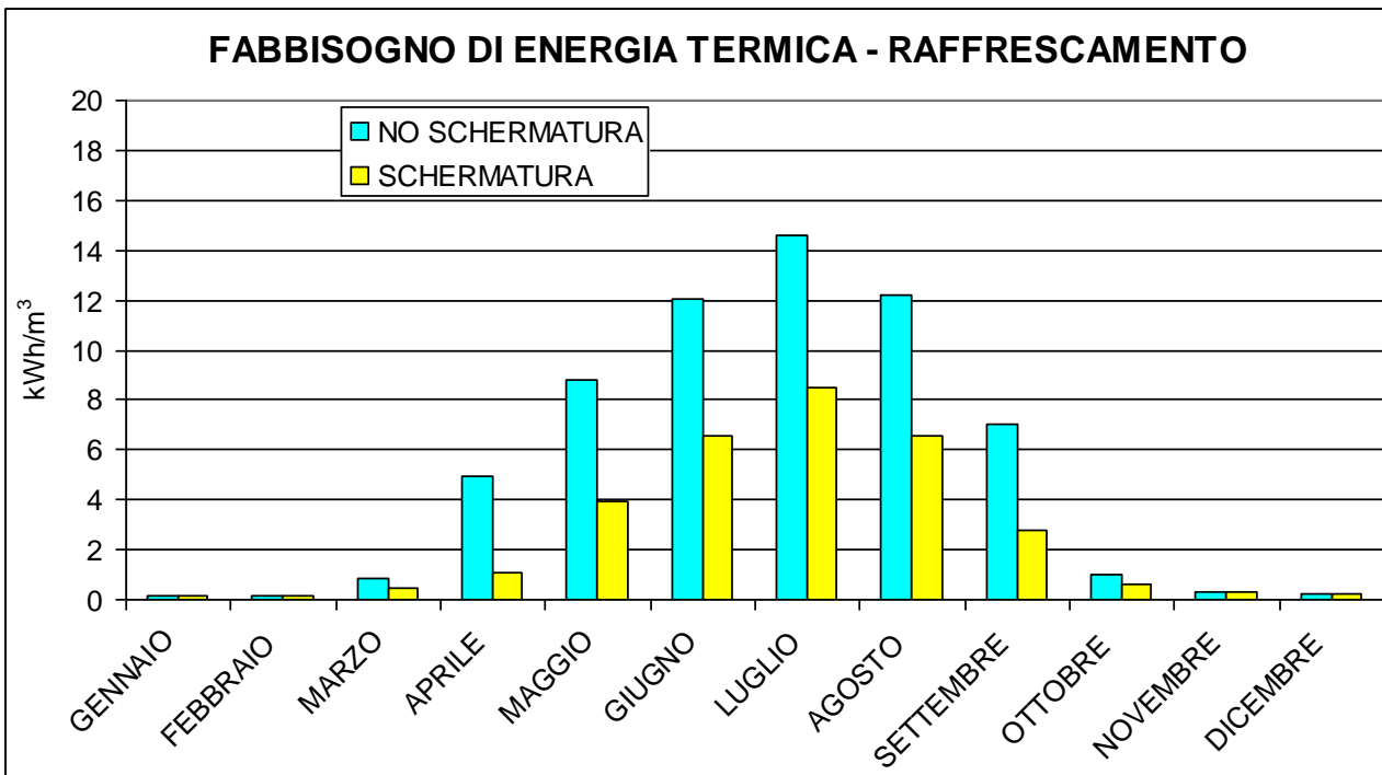
Figura 3.2.24 – Fabbisogno di energia termica per il raffrescamento, in presenza ed in assenza di schermature solari, per la città di Torino.
