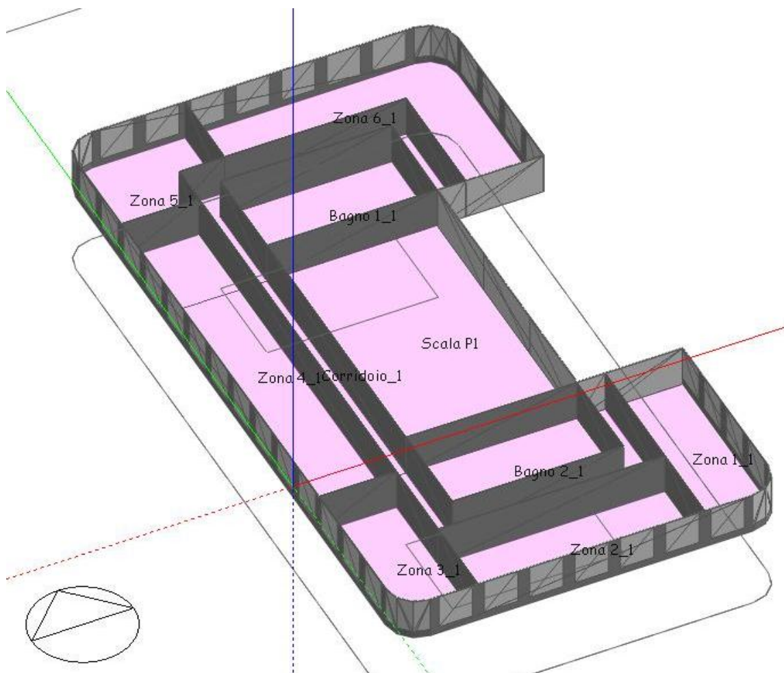
Figura 3.2.8 – Vista assometrica del 1° piano.
