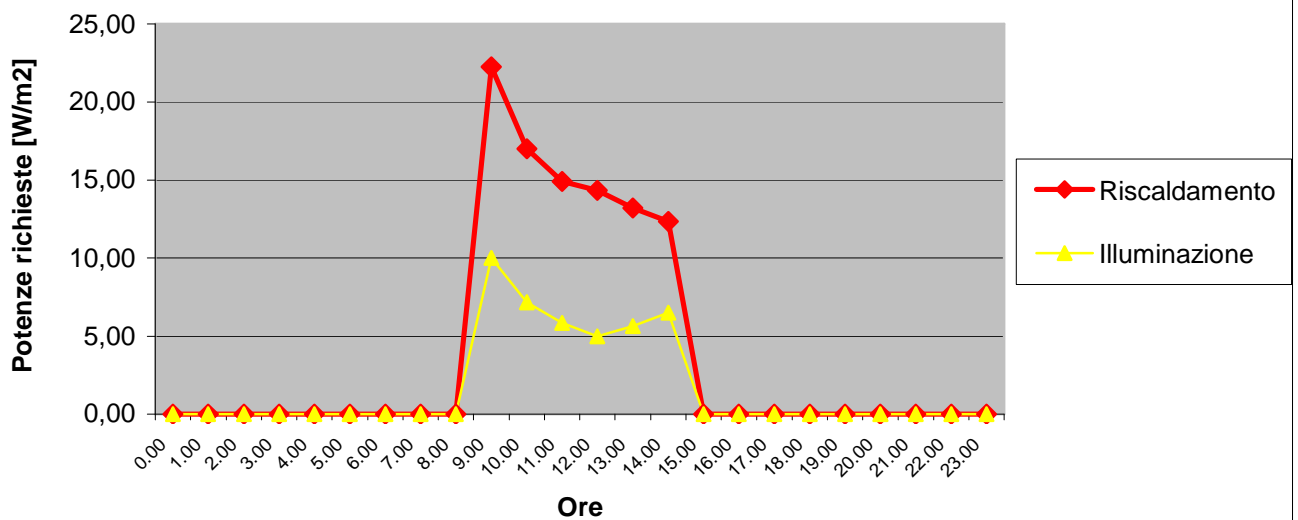
Profili di domanda energetica per riscaldamento ed illuminazione (giorno di progetto invernale: 21/12)
