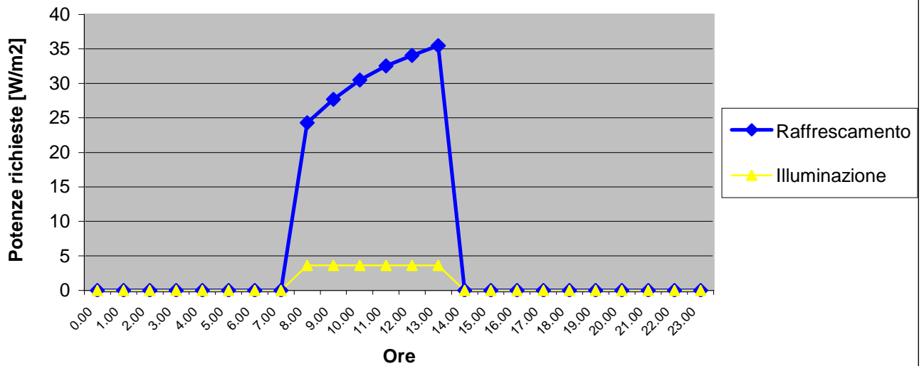
Profili di domanda energetica per raffrescamento ed illuminazione (giorno di progetto estivo: 21/06)
