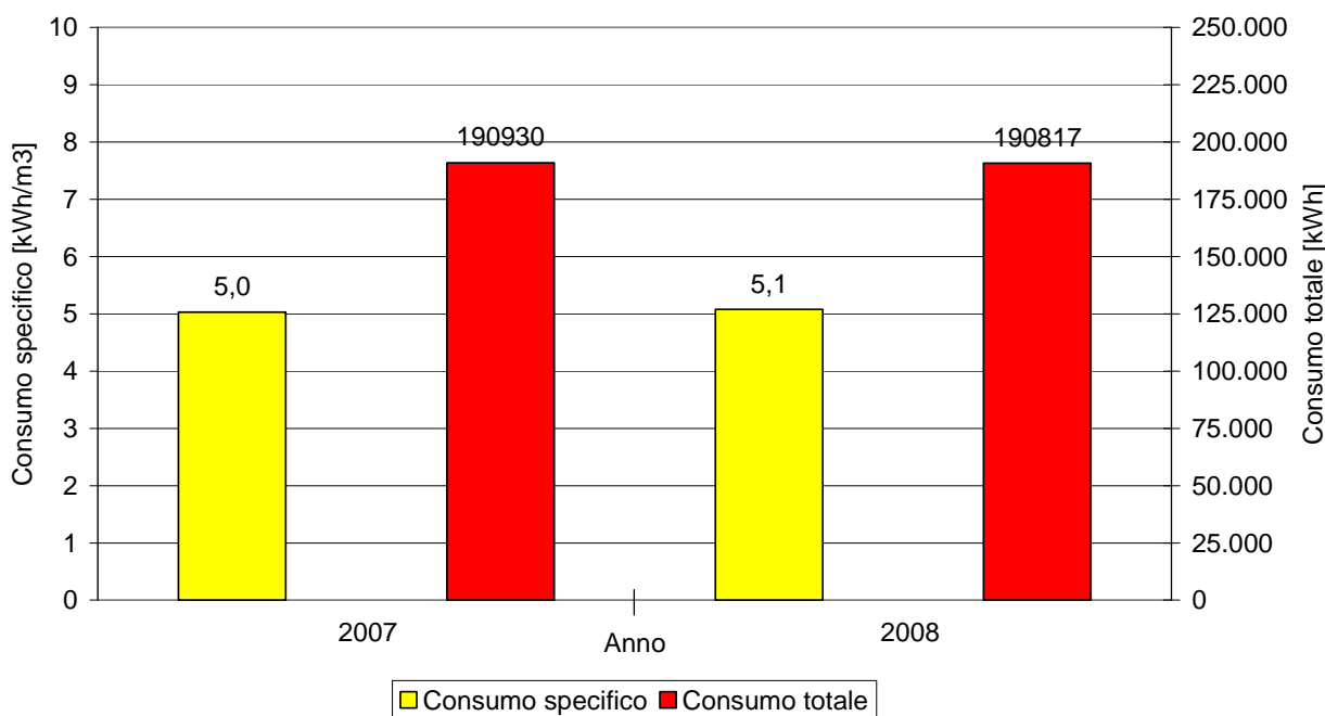
CONSUMO MEDIO TOTALE E SPECIFICO DI ENERGIA ELETTRICA NEI DUE ANNI DI ANALISI (43 edifici)
