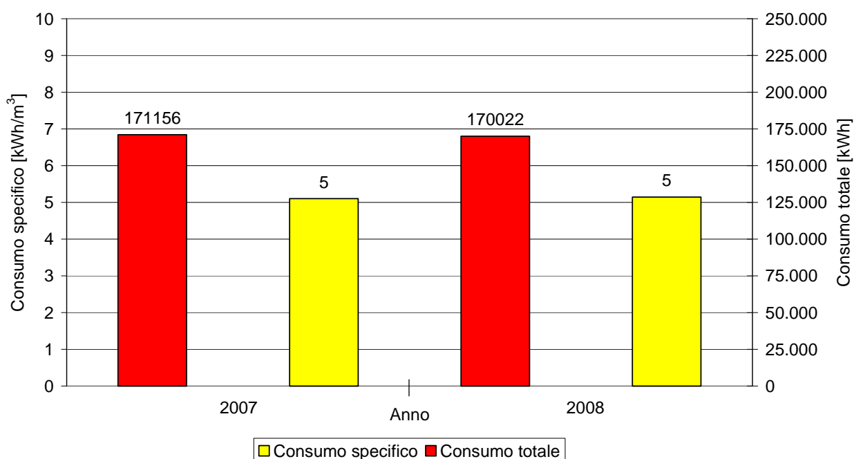
CONSUMO MEDIO TOTALE E SPECIFICO DI ENERGIA ELETTRICA NEI DUE ANNI DI ANALISI (29 edifici)
