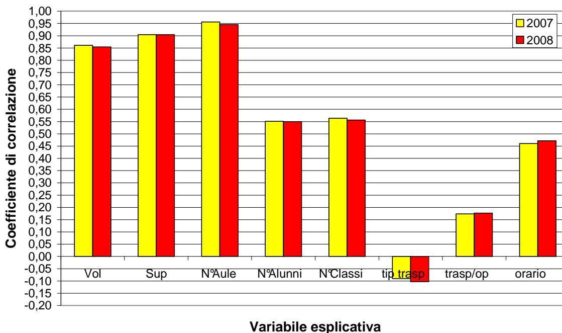
COEFFICIENTI DI CORRELAZIONE - CONSUMO ELETTRICO
