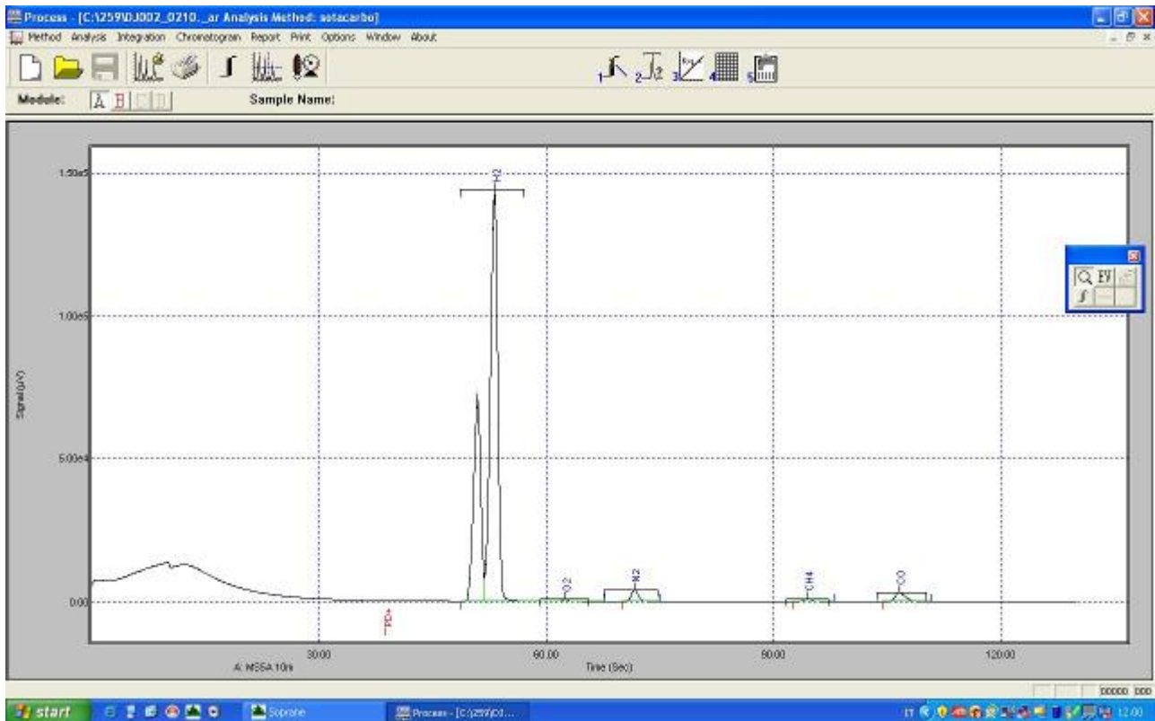
Figura 6 . Cromatogramma anomalo
