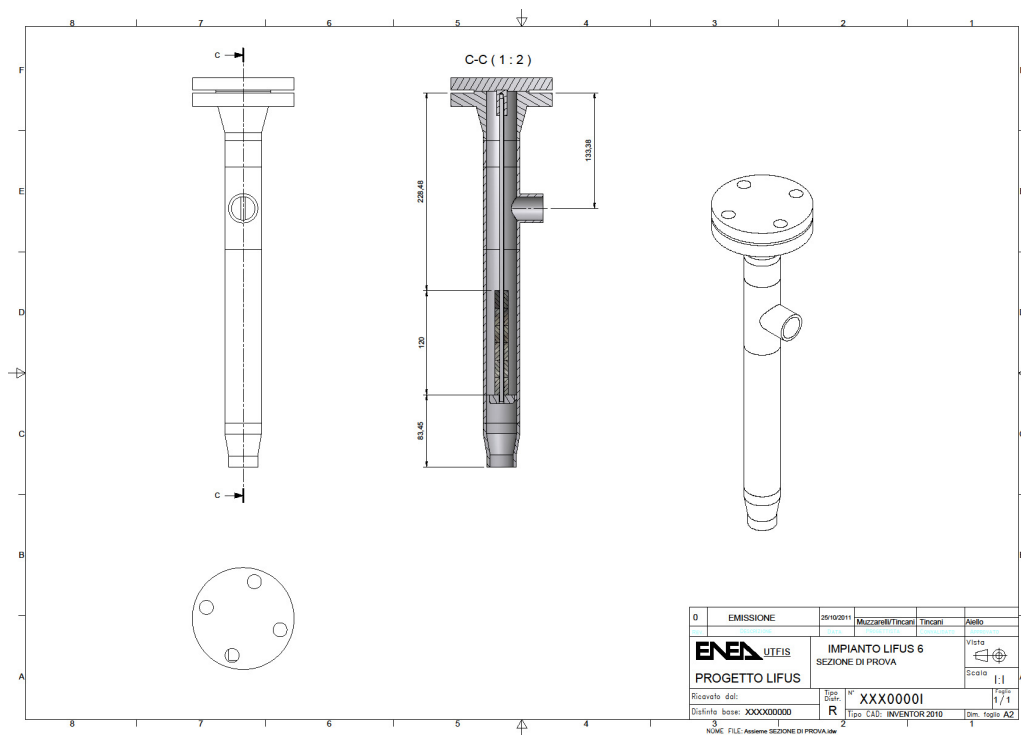
Figura 7: insieme della sezione di prova
