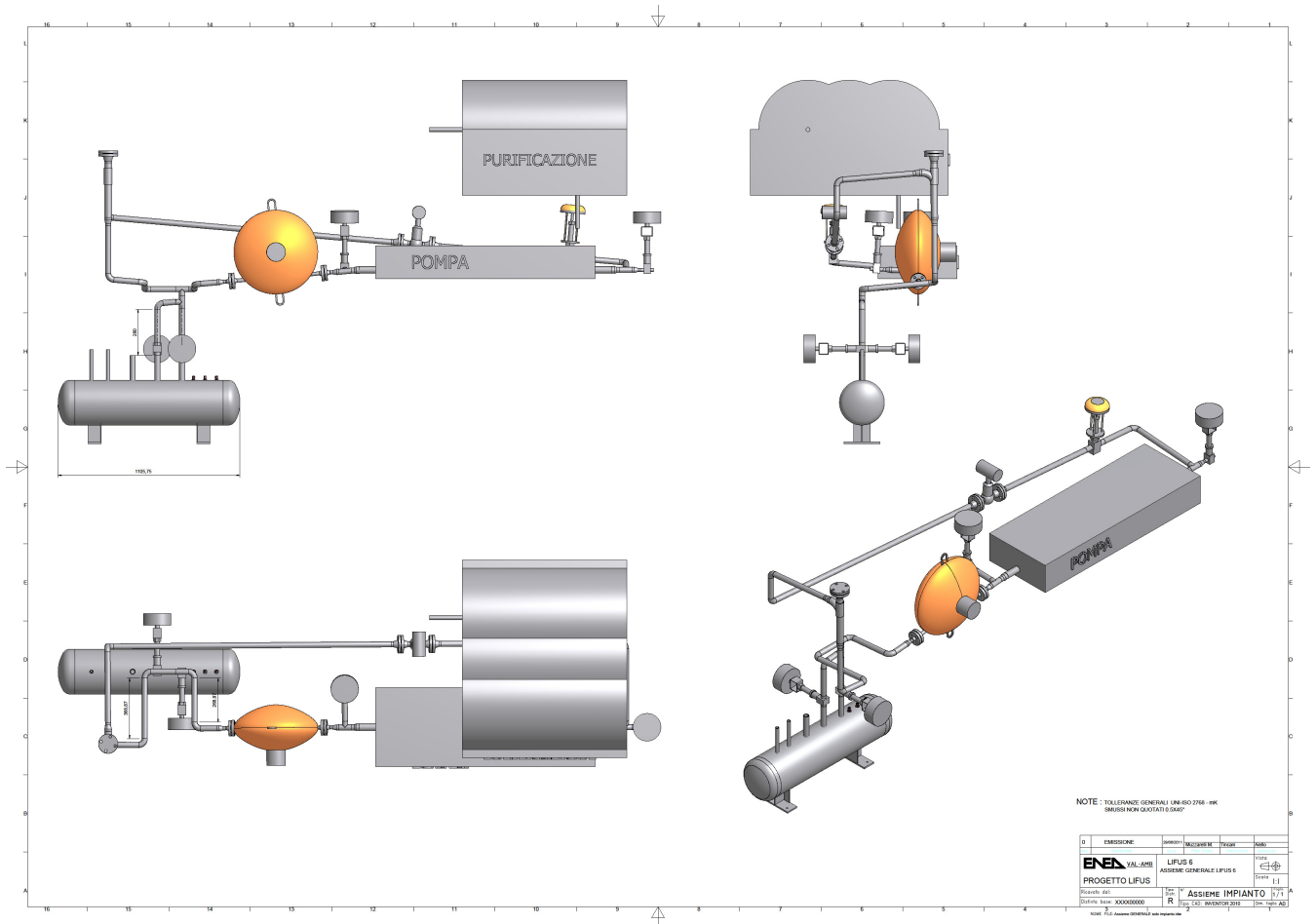
Figura 4: lay out generale dell'impianto
