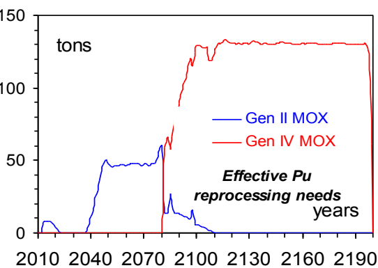
Figura 24: Riprocessamento Pu/Tipo-Reattore; Caso 1.
