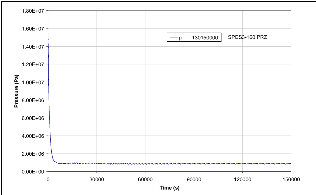
Fig.4.8 – SPES3-160 PRZ pressure
