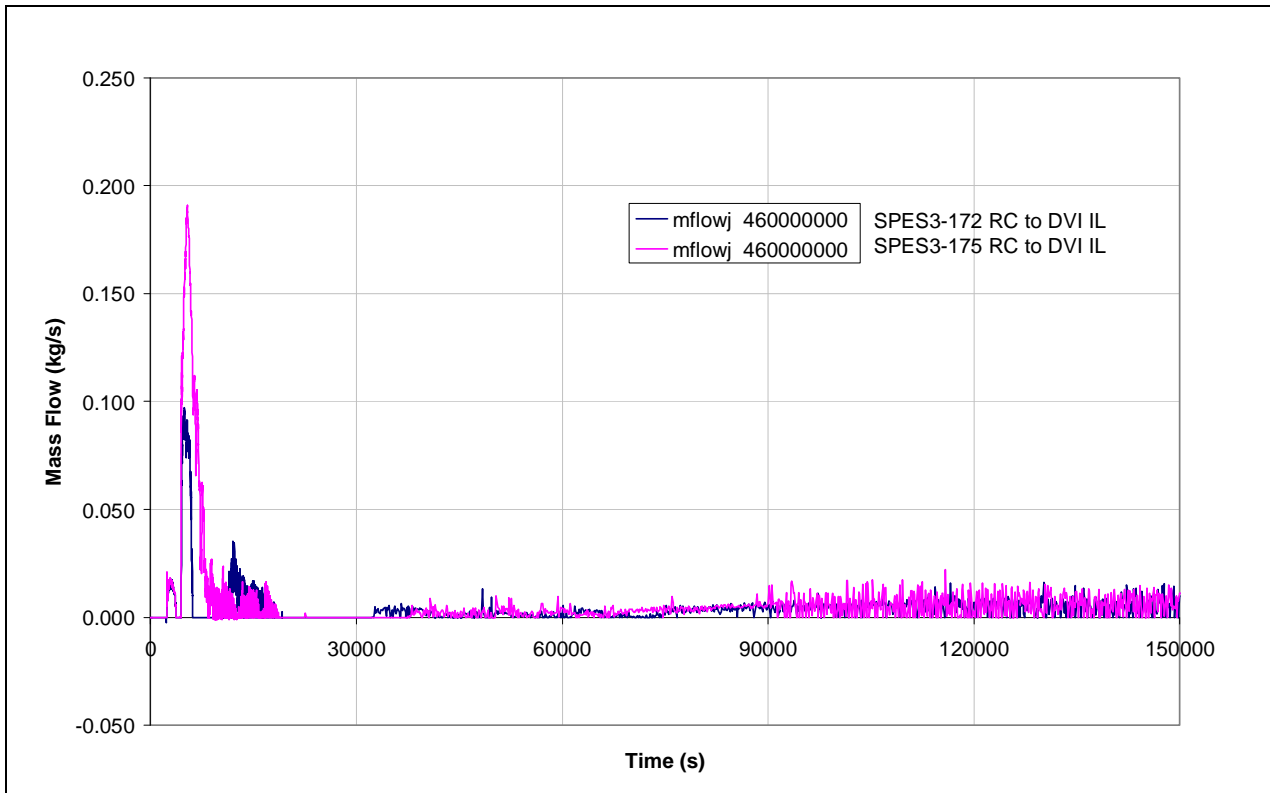
Fig.7. 57 - SPES3-172 and SPES3-175 RC to DVI mass flow IL
