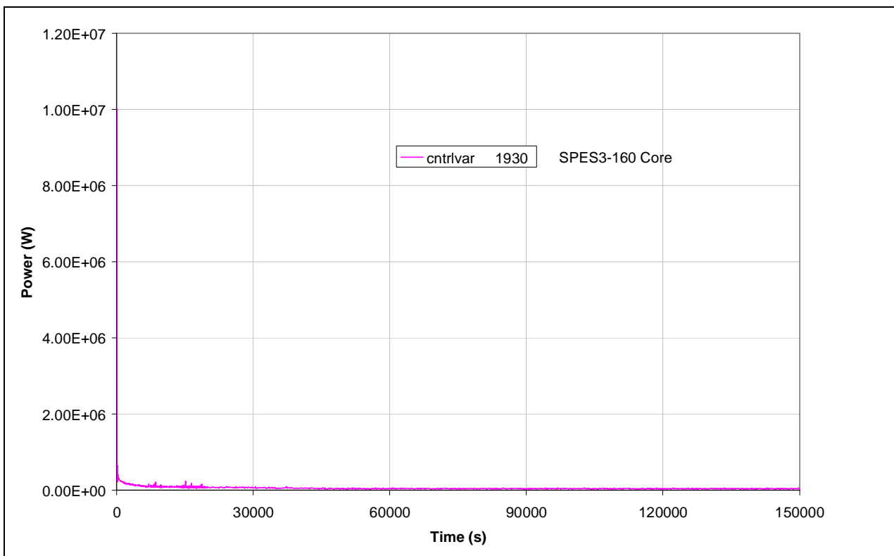
Fig.4.38 – SPES3-160 core power
