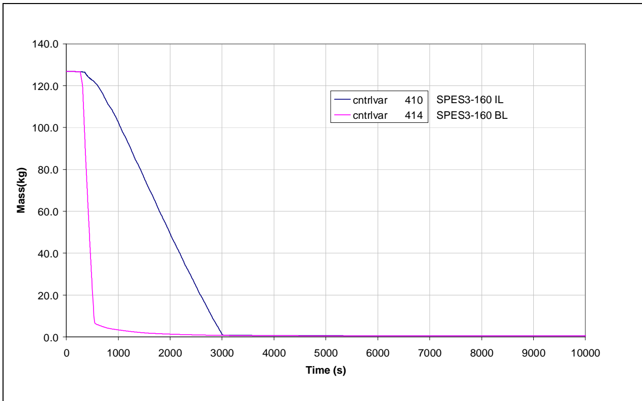
Fig.4.51 – SPES3-160 EBT mass
