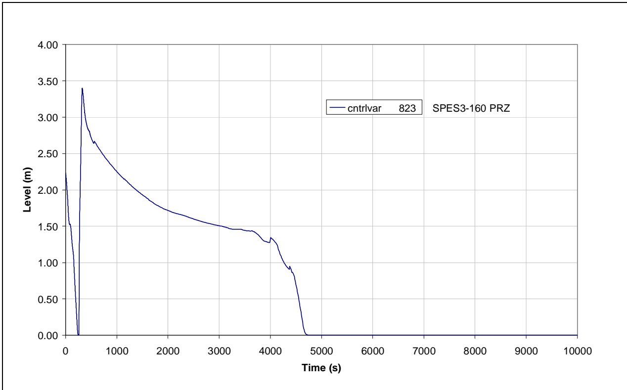
Fig.4.45 – SPES3-160 PRZ level
