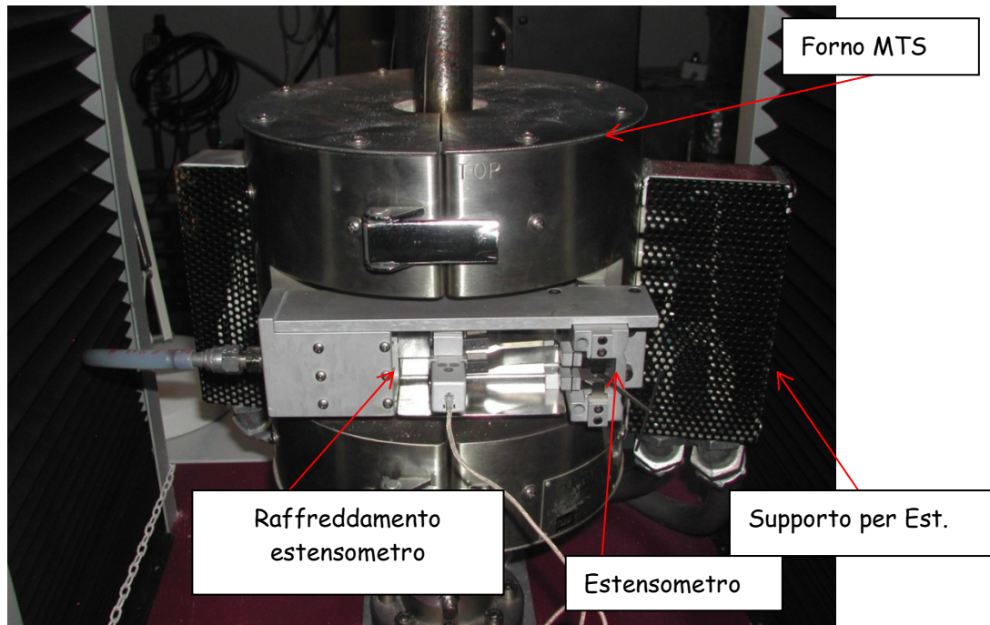
Figura 3: Forno e strumentazione di misura
