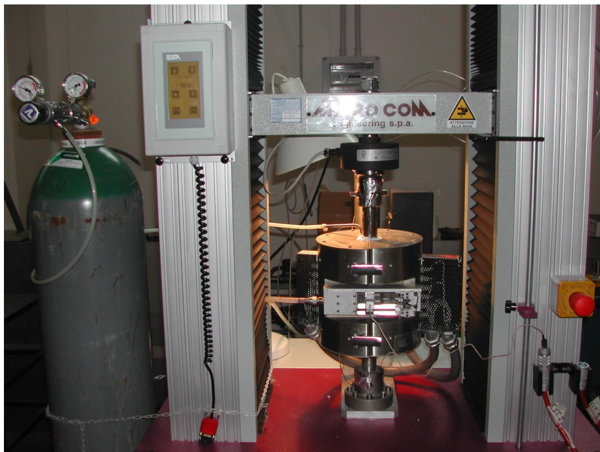
Figura 8: Configurazione di test completa
