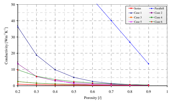
b)...porosity over 0.2
