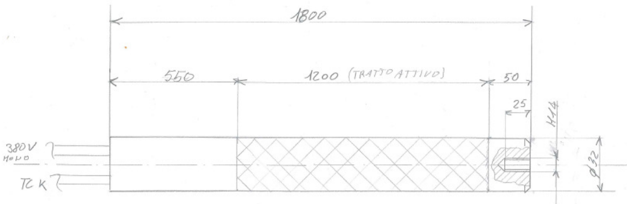
Fig. 53 – TxP design: PID.
