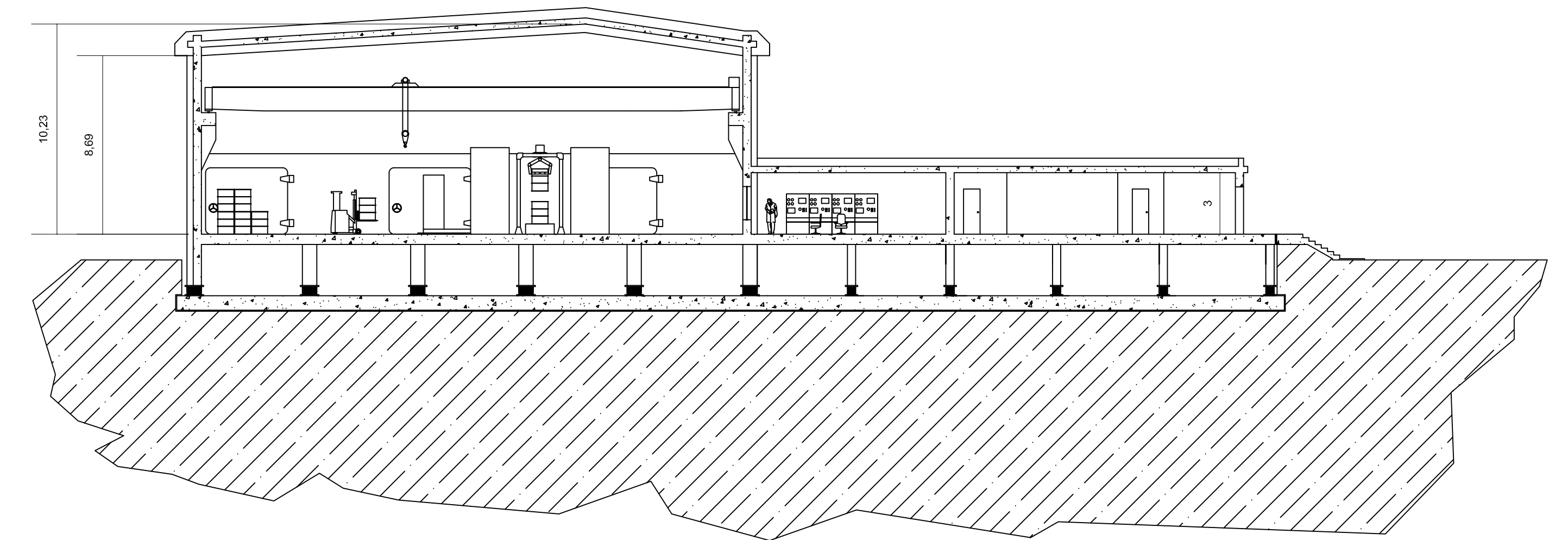
Sez. A-A
