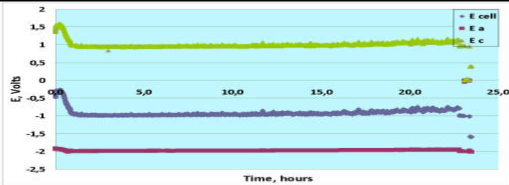
Andamento potenziali
