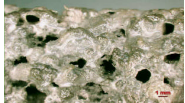
Deposito catodico
