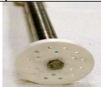
Disco di raccolta in allumina ( catch dish )
