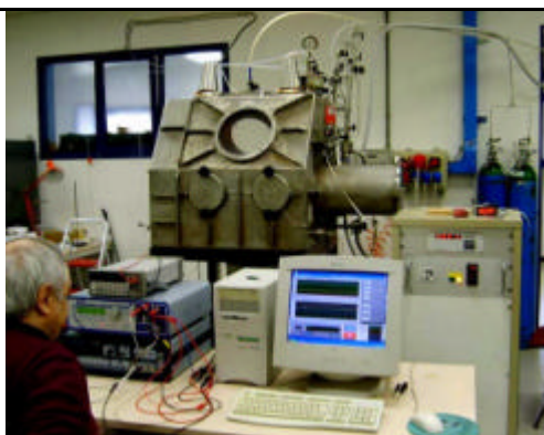
Figura 5 - Impianto pilota Pyrel II
