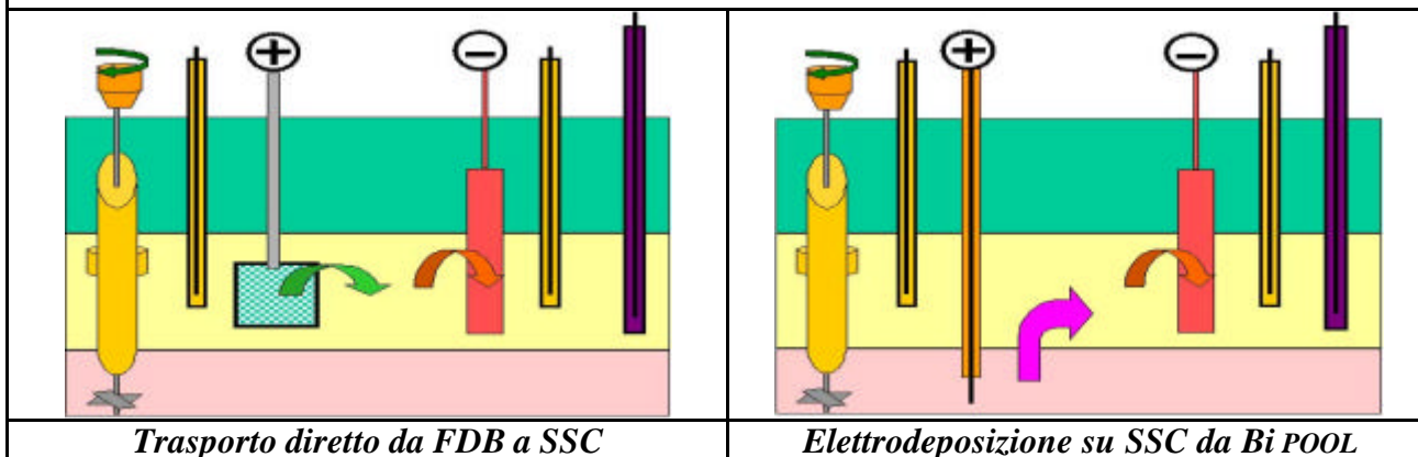
Figura 22 - Esperienze di elettrorefinazione
