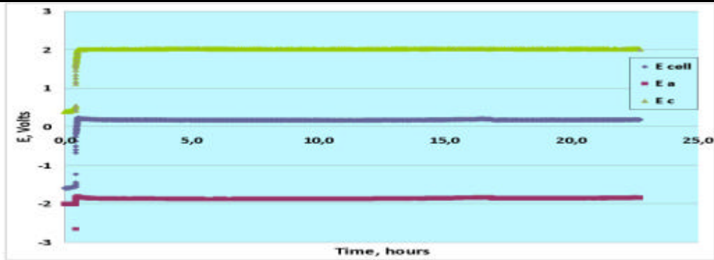
Andamento potenziali
