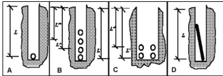
Figura 31 - Tipologie di scambiatori orizzontali. A) A tubo singolo; B) A tubi multipli sovrapposti; C) A tubi multipli affiancati; D) A spirale 25 .
