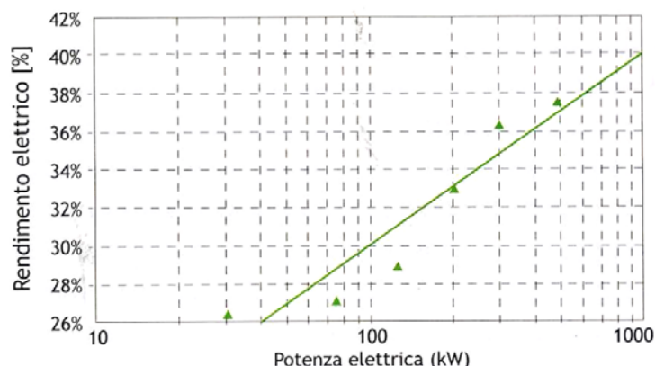
Figura 63 – Rendimento elettrico in funzione della taglia per alcuni MCI. Fonte: E. Macchi, S. Campanari, P. Silva, La microgenerazione a gas naturale , 2005, Polipress, Milano.
