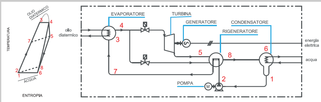
Figura 24 – Schema di funzionamento del ciclo ORC. Fonte:www.turboden.it
