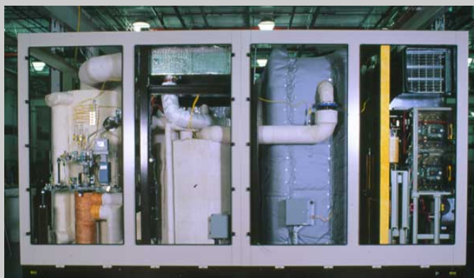
Figura 51 - Esempio di celle ad acido fosforico.
