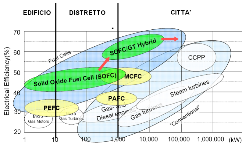
Figura 43 - Campi di applicazione per i diversi impianti di cogenerazione (GTT – European Fuel Cell Conference).
