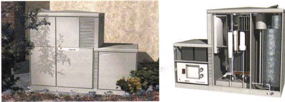
Figura 54 – Impianto GE HomeGen (Ge Microgen – Plug Power) da 7 kW el . Fonte: E. Macchi, S. Campanari, P. Silva, La microgenerazione a gas naturale , 2005, Polipress, Milano.
