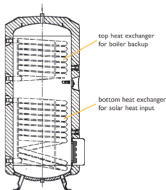
Figura 16 - Struttura e aspetto esterno di un serbatoio di accumulo per impianti solari termici.
