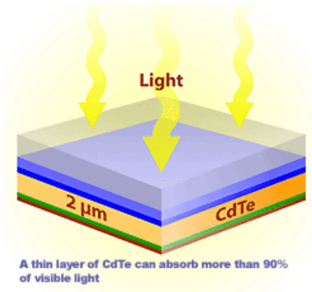
Figura 5 - Struttura di una cella al telloruro di cadmio.
