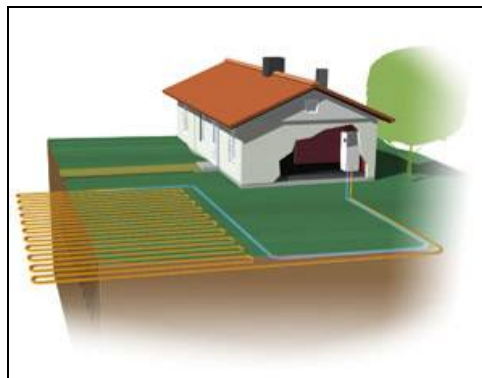
Figura 30 - Schema di funzionamento di un impianto con scambiatore orizzontale per terreno 24 .
