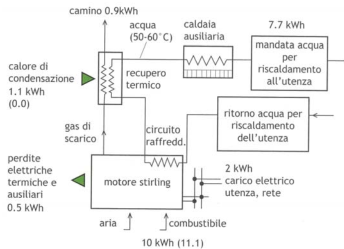
Figura 67 – Esempio di schema di impianto di un sistema cogenerativo a motore Stirling. I bilanci energetici si riferiscono ad una unità con rendimento elettrico pari al 20%. Fonte: E. Macchi, S. Campanari, P. Silva, La microgenerazione a gas naturale , 2005, Polipress, Milano.
