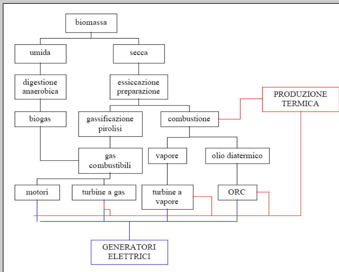
Figura 19 - Possibile suddivisione delle modalità di produzione di energia da biomasse.
