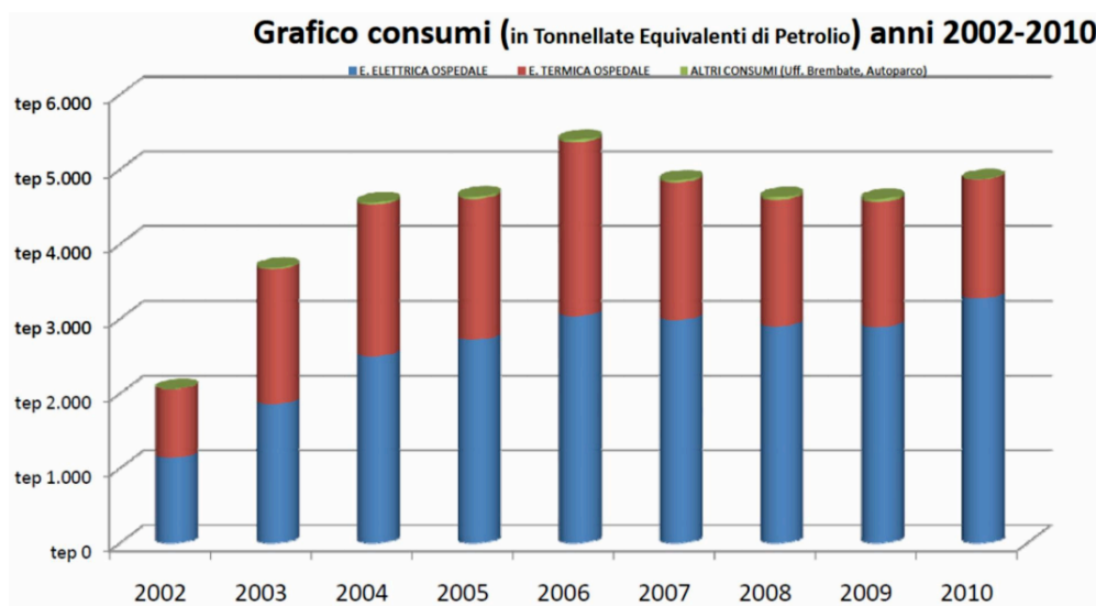
Figura 35: andamento dei consumi totali di energia Sant'Andrea [39]
