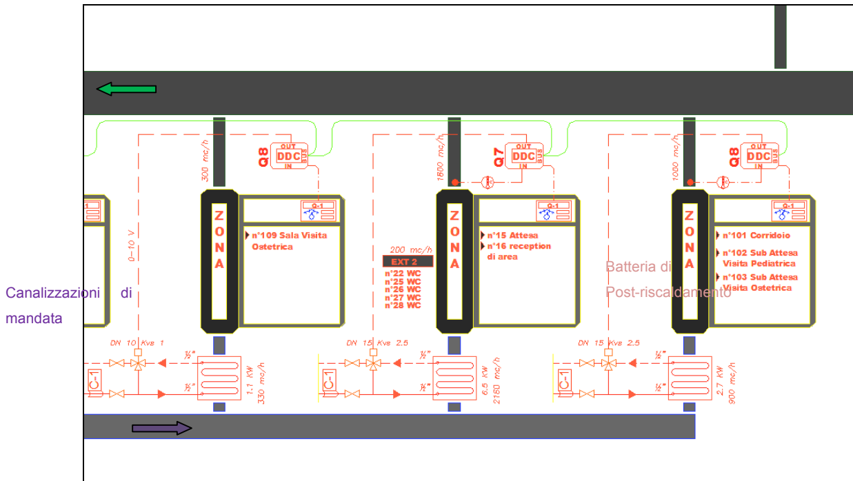
Figura 39: schema funzionale zone con condizionamento a tutta aria.
