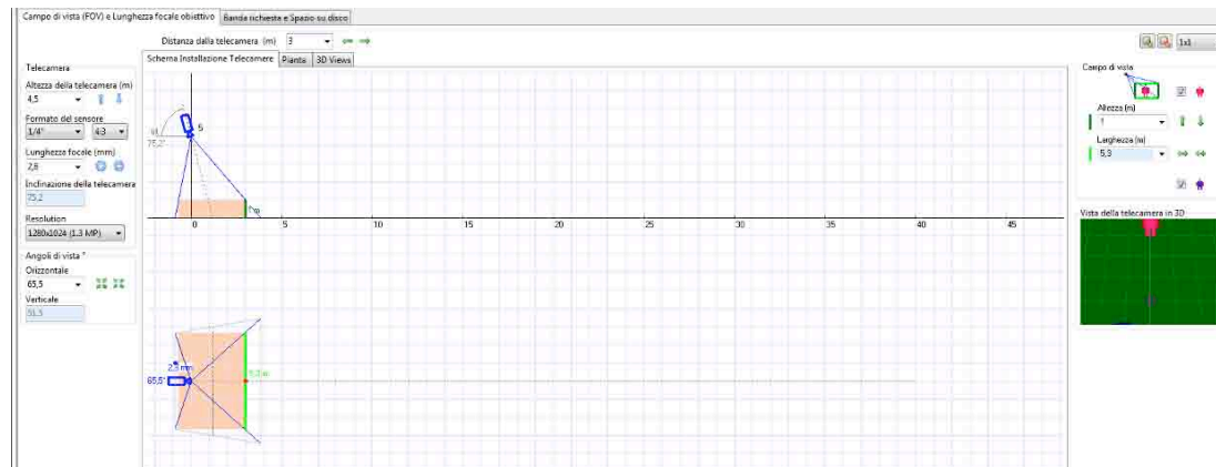
Figura 42: Configurazione Modulo EyeSense scenario Predicting situazione marciapiede
