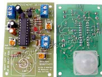
Figura 31: esempio di integrazione di un sensore PIR, un sensore crepuscolare LDR e un sensore di movimento IC
