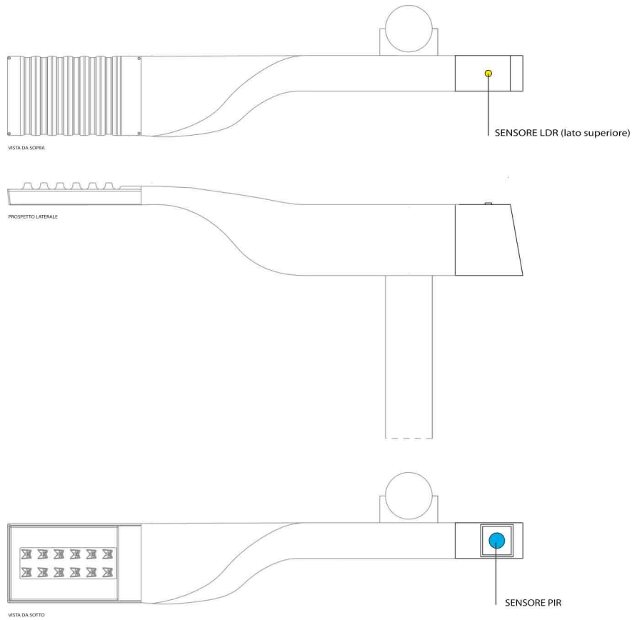
Figura 35: Integrazione verticale del modulo PreSense rispetto all'apparecchio PLUS
