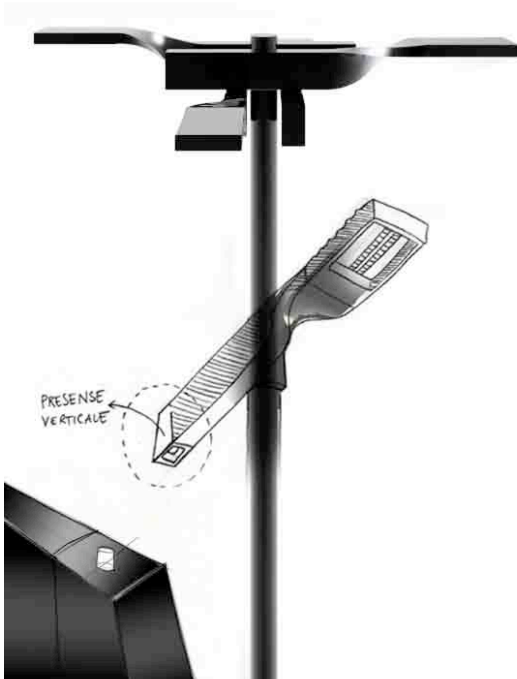
Figura 37: Immagine che illustra la configurazione in cui il sistema PLUS integra il Modulo PreSense verticale
