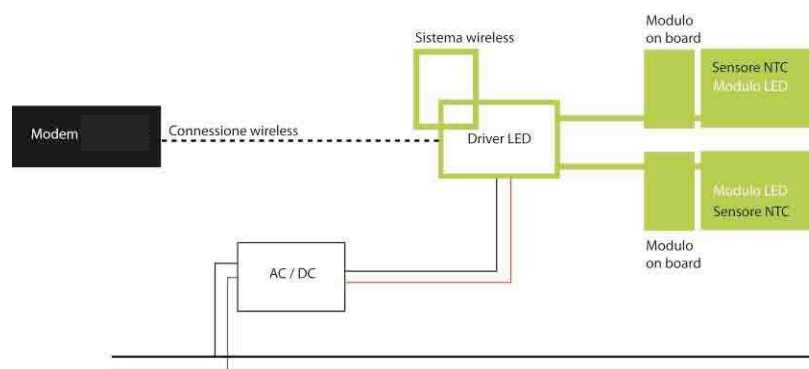
Figura 21: Sistema di connessione wireless
