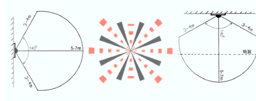
Figura 30: angoli di rilievo
