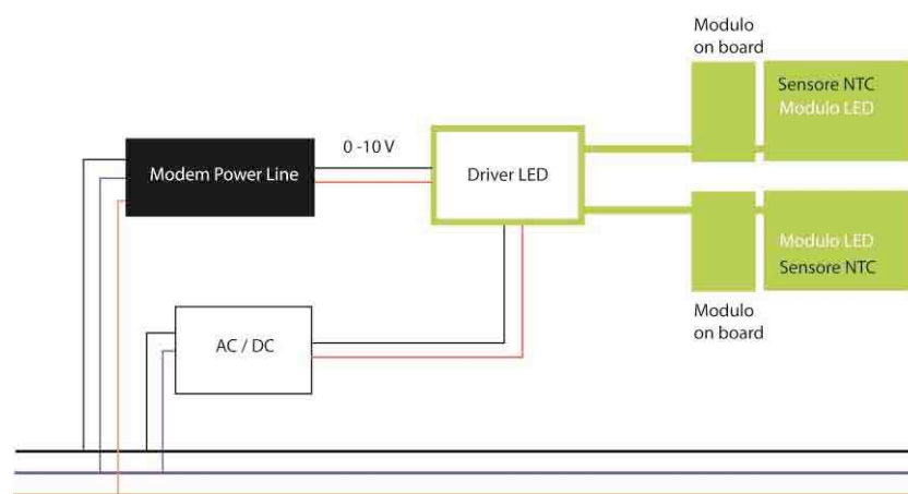
Figura 20: Sistema di connessione cablato
