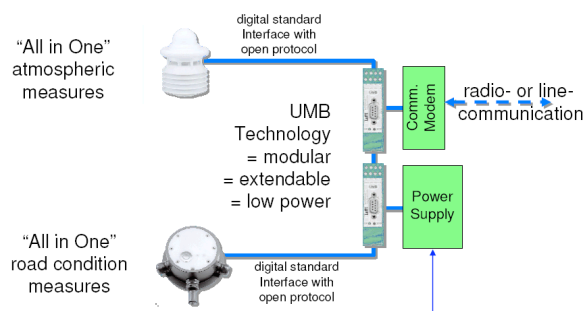
Figura 28: Sistema di comunicazione dei sensori
