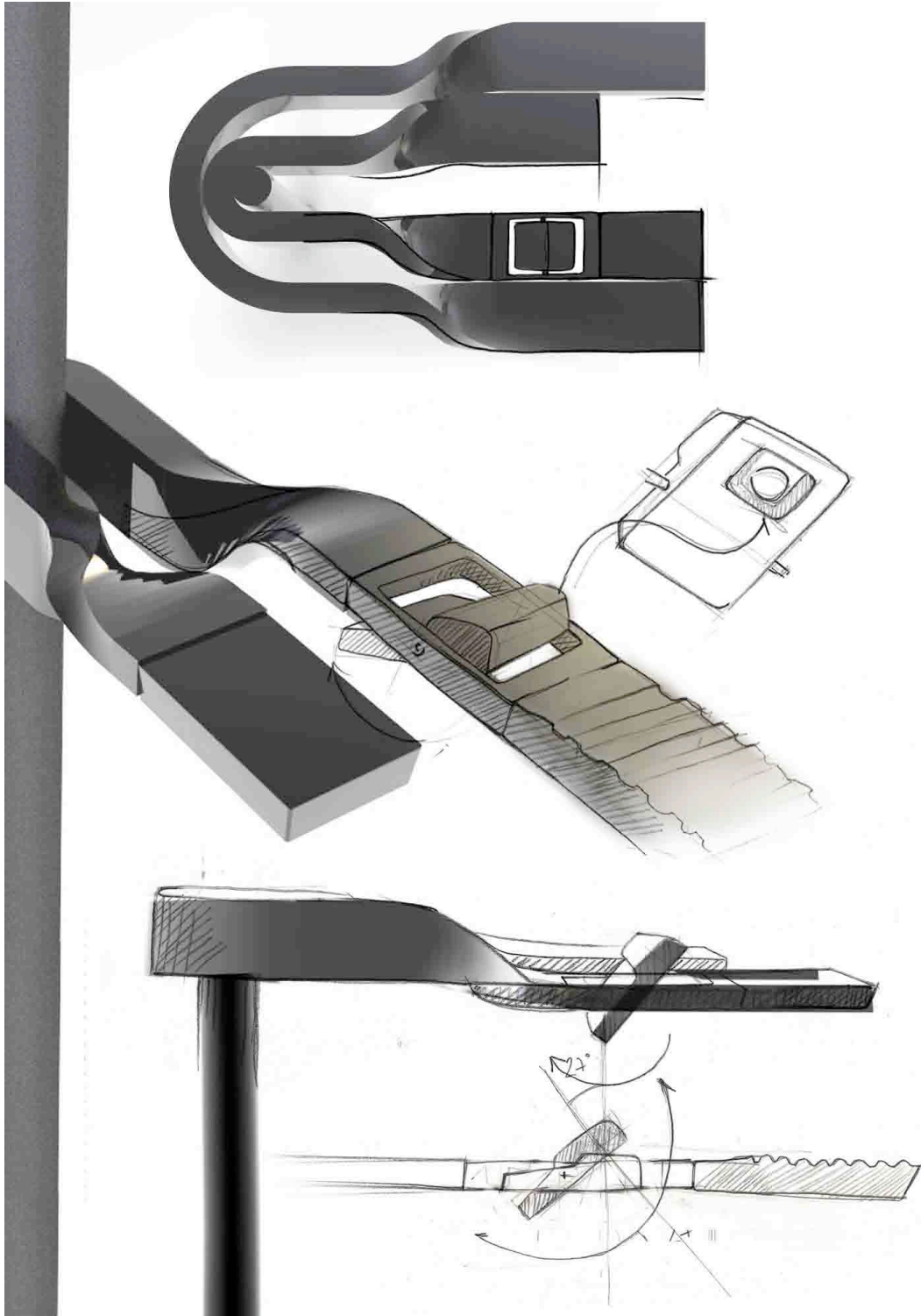
Figura 41: Immagini di rendering che illustrano l'integrazione della videocamera rispetto al sistema di illuminazione PLUS
