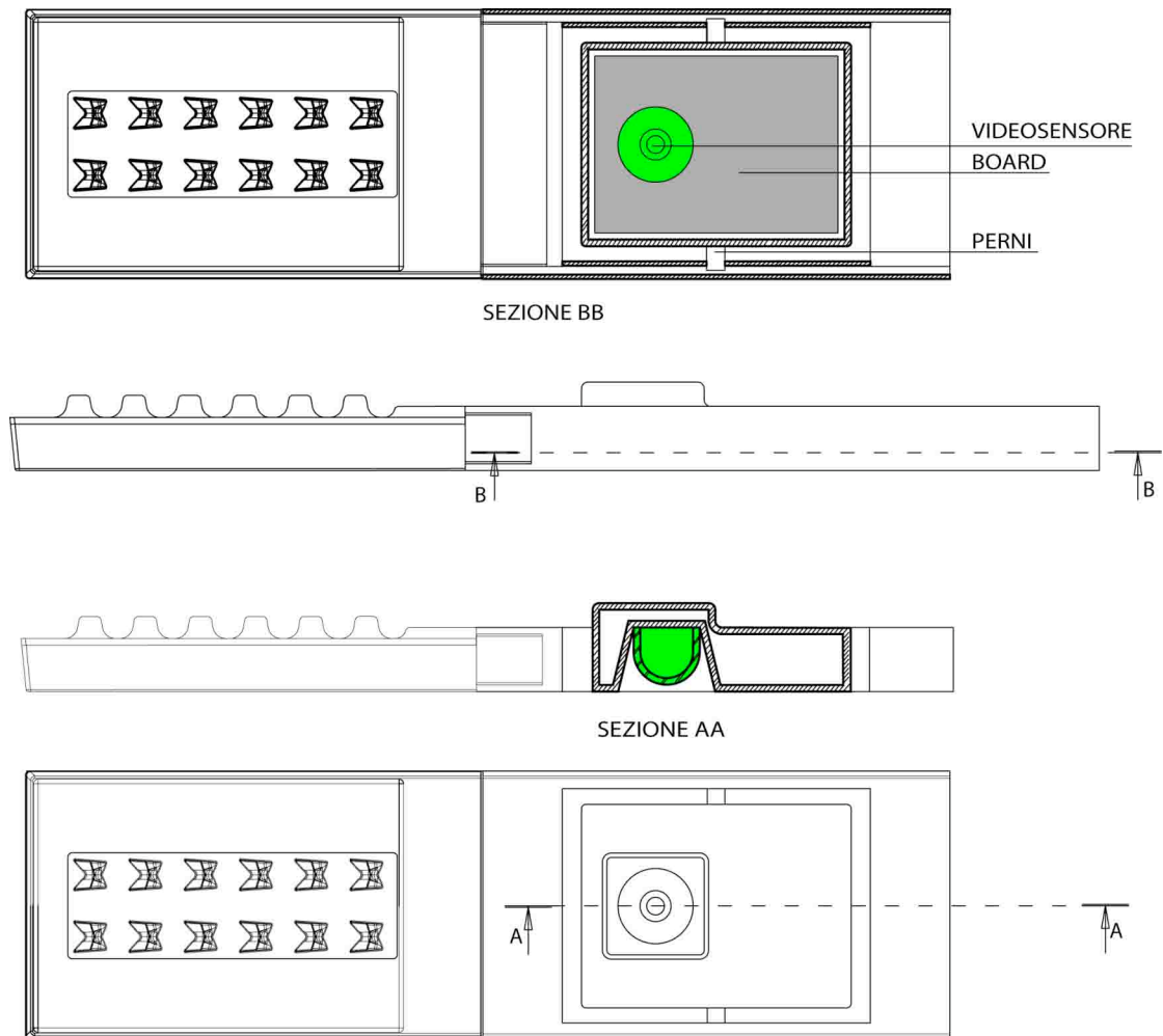
Figura 40: Configurazione del video sensore e sistema di perni di rotazione che permettono l'inclinazione della videocamera
