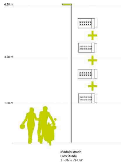
Figura 25: configurazione dell'apparecchio di illuminazione PLUS per strade a traffico misto
