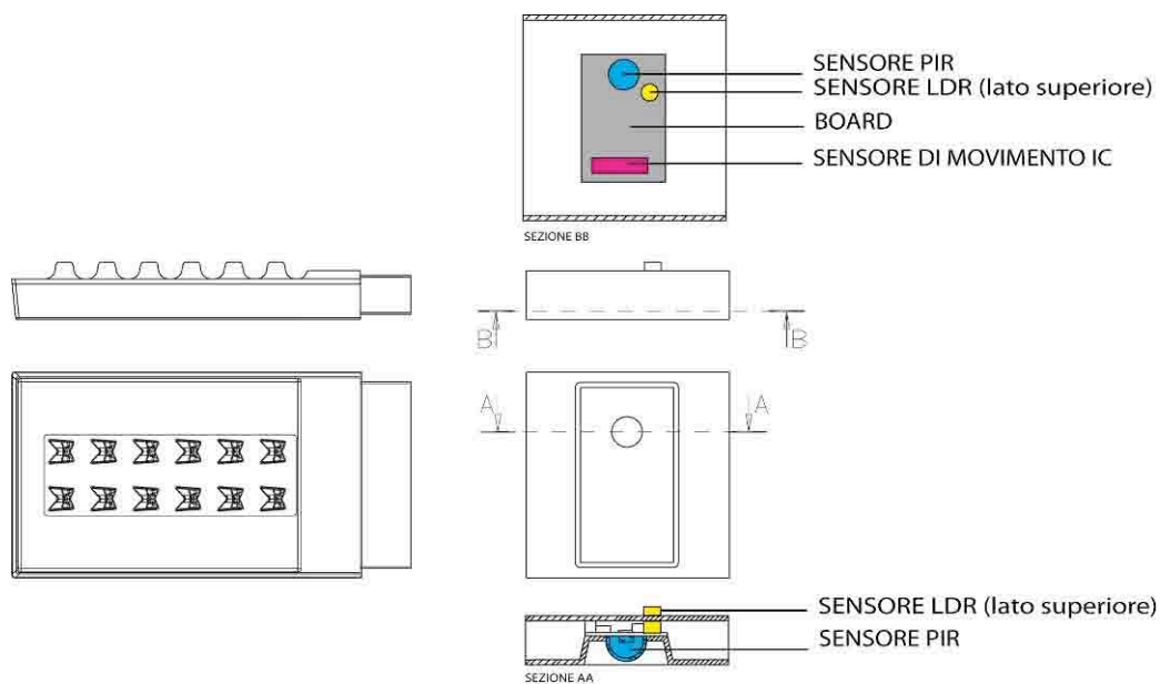
Figura 33: Modulo PreSense e sensori integrati
