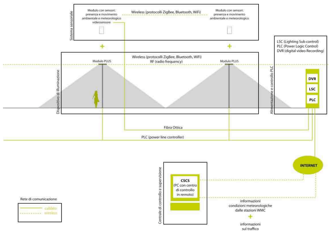
Figura 19: Architettura del sistema di Smart Lighting
