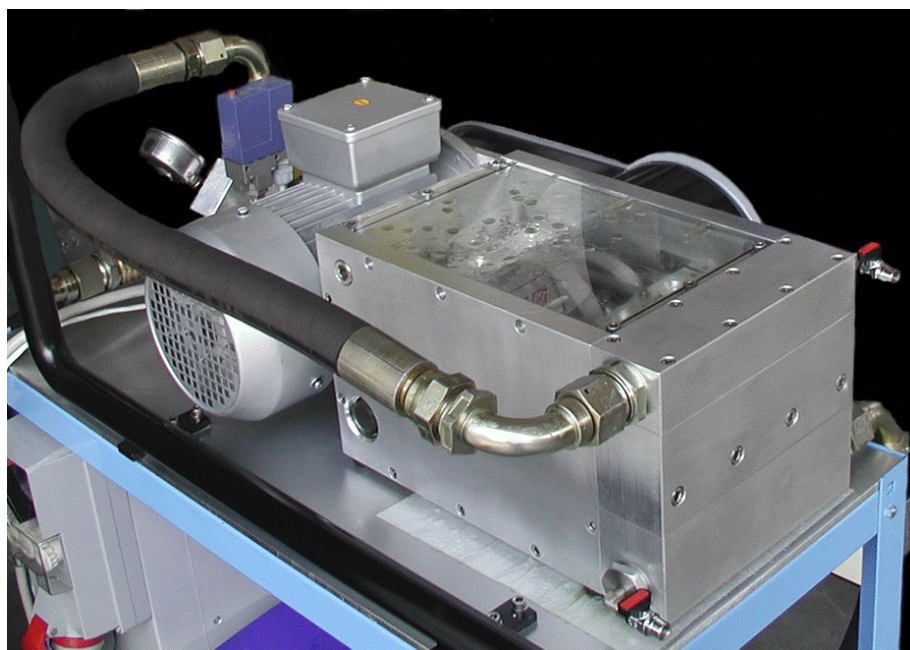
Figura 25. La nuova pompa Triplex a flusso continuo (1 m 3 /h, 30 Bar, motore da 1.1 kW)
