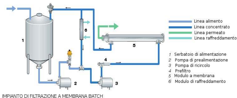
Figura 13. Schema di impianto pilota batch
