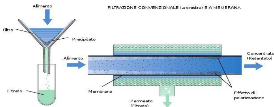
Figura 3. Sistema di filtrazione perpendicolare e tangenziale
