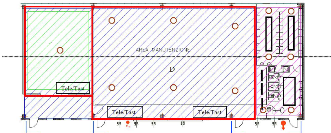
Figura 5 Disposizione sensori, dispositivi di controllo (telecomando-Tastiera), pulsanti-parte 3
