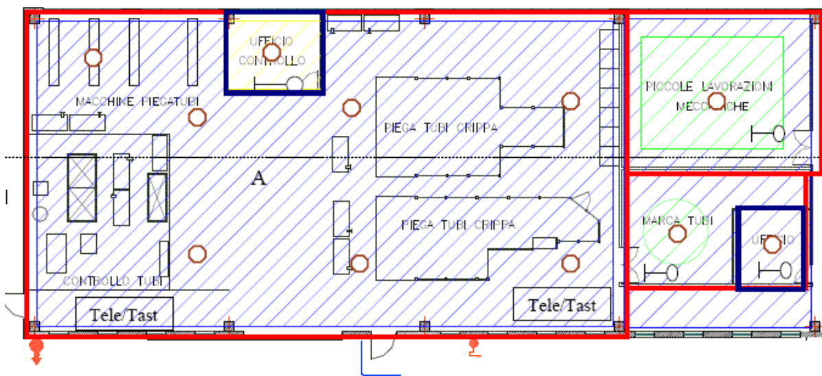
Figura 3 Disposizione sensori, dispositivi di controllo (telecomando-Tastiera), pulsanti-parte 1
