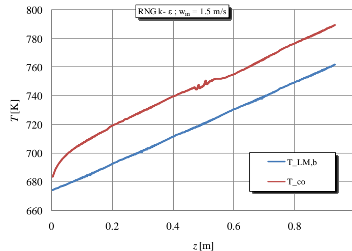
Andamento temperatura di bulk e di camicia in funzione della coordinata assiale ( RNG K-ε e RSM)
