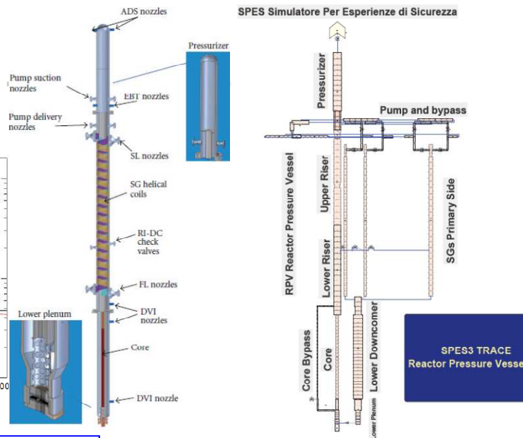
Fig. 4-2: Nodalizzazione del sistema primario di SPES-3.
