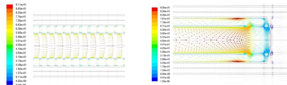
Fondo del canale con aria
