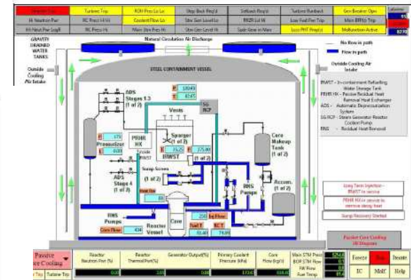
schiera relativa ai sistemi di sicurezza di emergenza per il raffreddamento del core.
