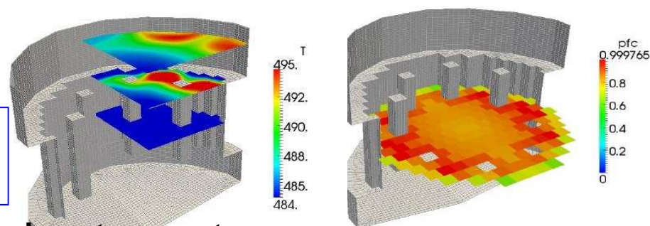
Distribuzione temperatura
