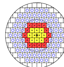
Distribuzione combustibile core
