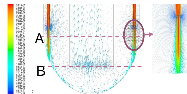
Analisi del campo di velocità
