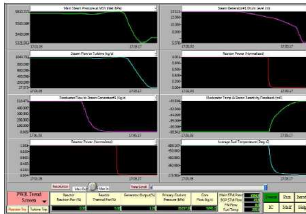
3. Maschera relativa al circuito primario e ad alcuni controlli considerati dal simFig. 7. Andamento temporale di alcune grandezze significative durante il transitorio che segue alla chiusura delle valvole di alimentazione dei generatori di vapore.
