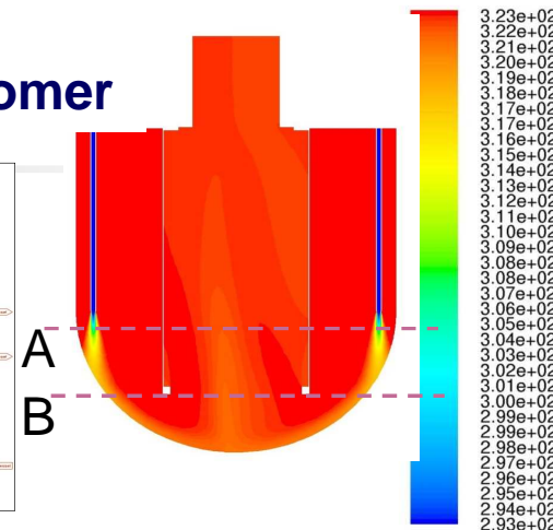
Analisi del campo di Temperatura
