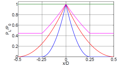
Potenza trasferita vs. x/D per Xt/D=1 (verde), 3/4 (viola), 1/2 (rosso), 1/4 (blu).
