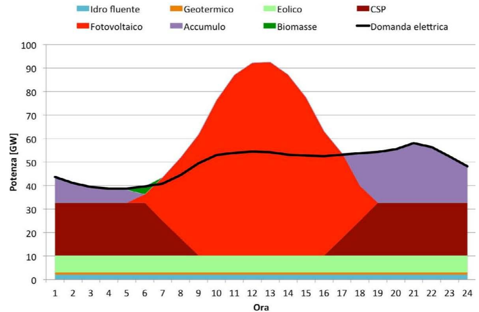
Carico e generazione oraria estiva nello scenario Blue 100% FER
