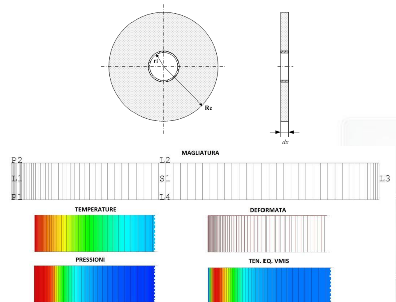
Studio termo meccanico di un elemento di accumulo di calore
