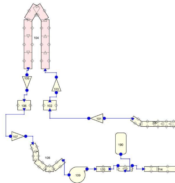
Esempio di nodalizzazione con RELAP5-3D
