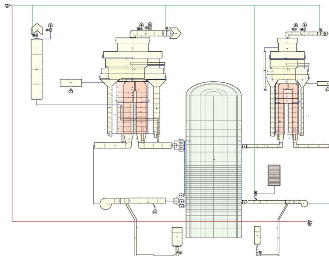
Esempio di nodalizzazione con RELAP5-3D
