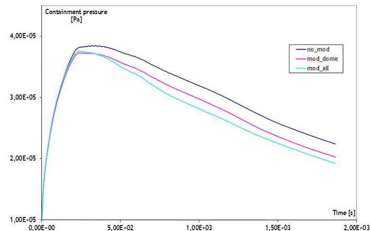
Esempio di andamenti della pressione del contenimento
