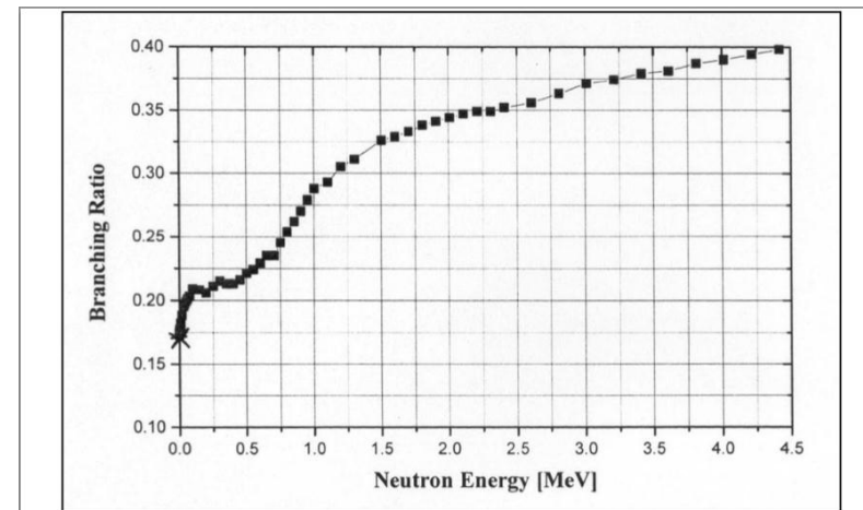
Figura 6: Probabilità di formazione dello stato meta stabile ^{242m}\text{Am} a seguito della reazione (n, \gamma) su ^{241}\text{Am} in funzione dell'energia dei neutroni [19].
