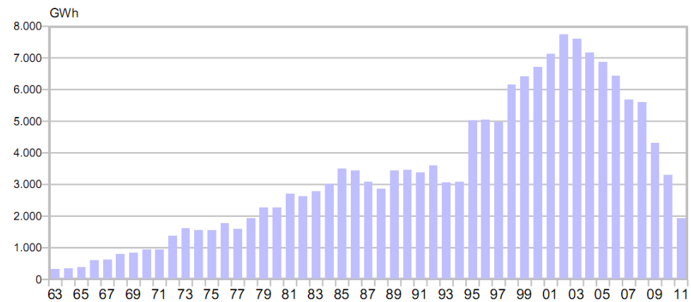
Andamento della potenza da pompaggio utilizzata (Terna, dati e statistiche)
