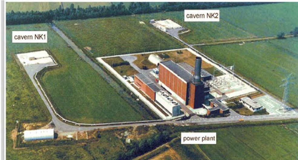
Impianto CAES di Huntorf (Germania)
