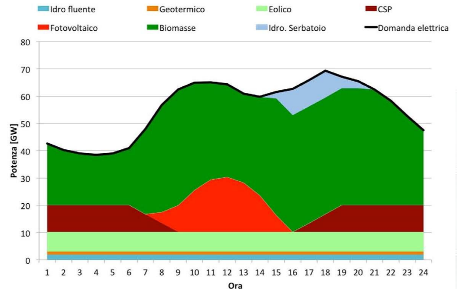
Carico orario invernale, scenario Blue 100% FER
